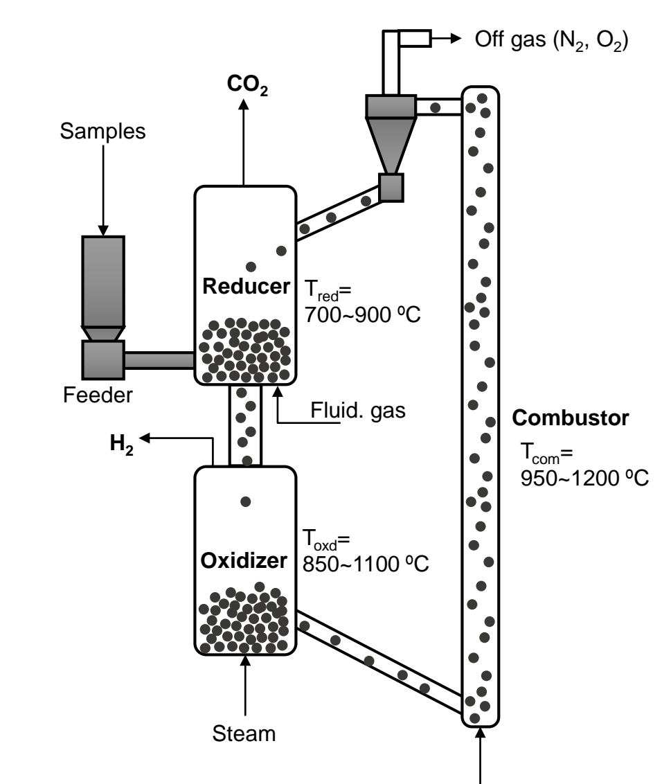
CO 2 フリー水素製造システム
