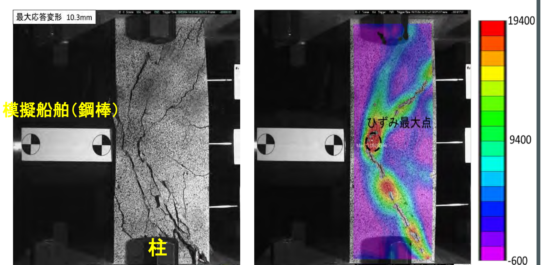
鉄筋コンクリート造柱への模擬船舶の衝突実験
