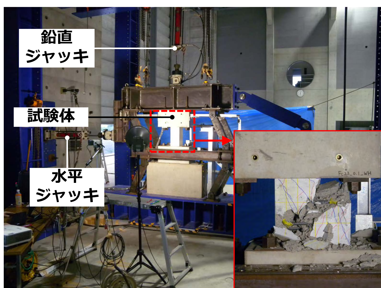
加力装置および軸崩壊後の試験体の様子
