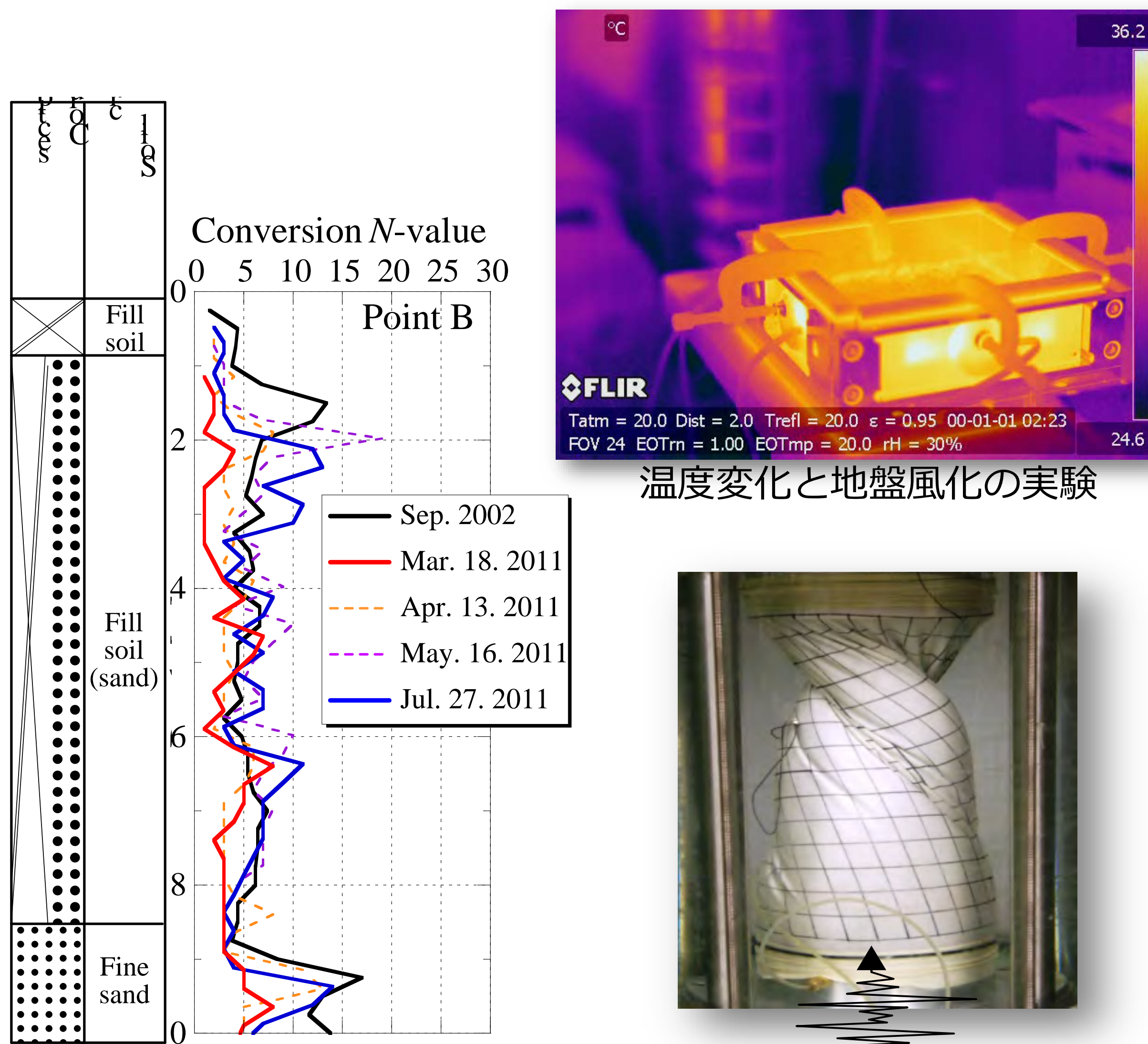
液状化発生前後の地盤強度の変化と中空筒試体による液状化実験
