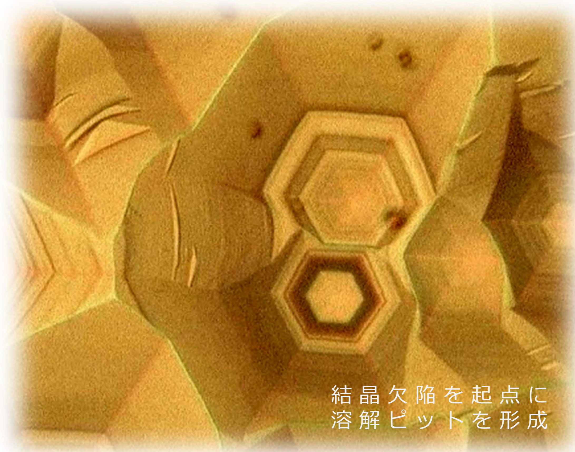
SiCが溶解する様子(1300℃)
