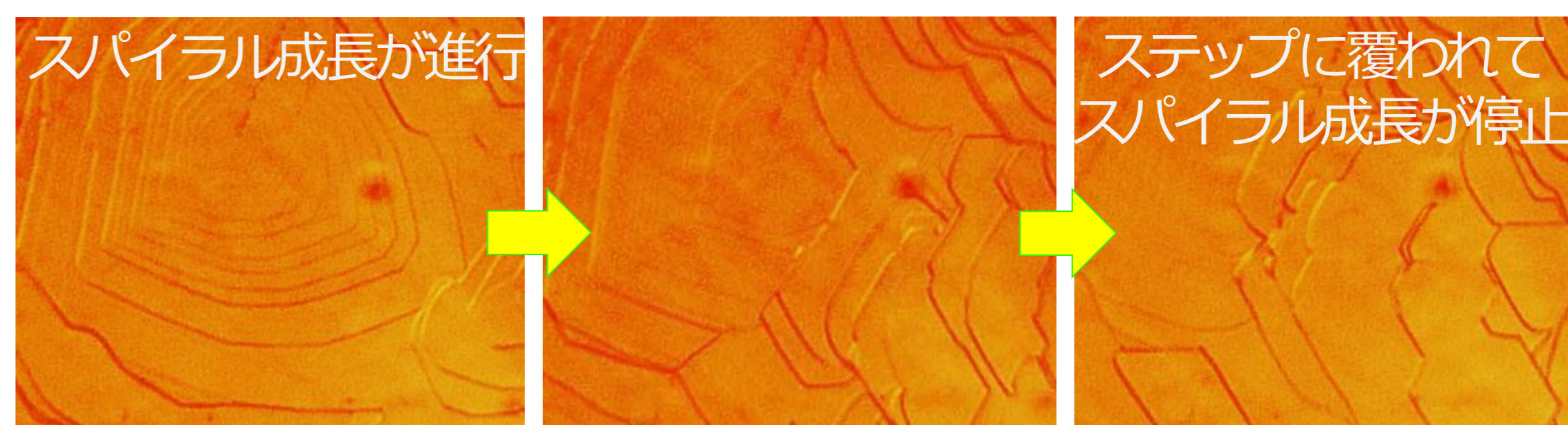
SiCが成長する様子(1400℃)
