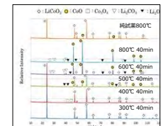
加熱後の正極材のXRDスペクトル
