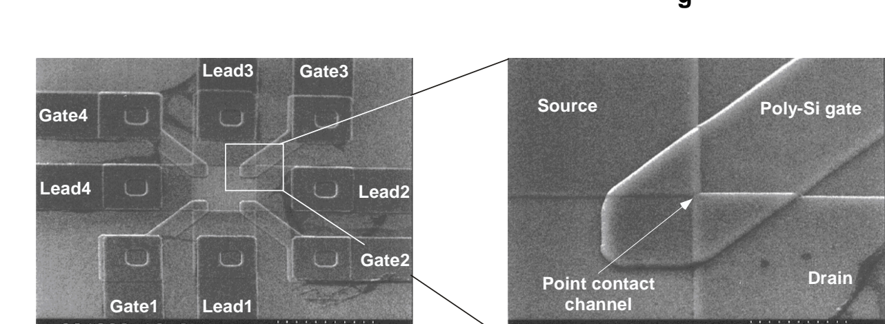
Fig. 4. Beyond CMOSの一種である室温動作の単電子トランジスタの集積化とCMOSとの融合に世界で初めて成功。
