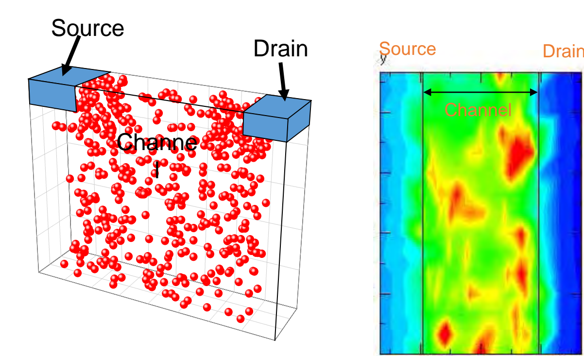
Fig. 2. トランジスタのさらなる微細化を阻害する分散不純物によるランダムな特性ばらつきを実測評価し改善策を提案。
