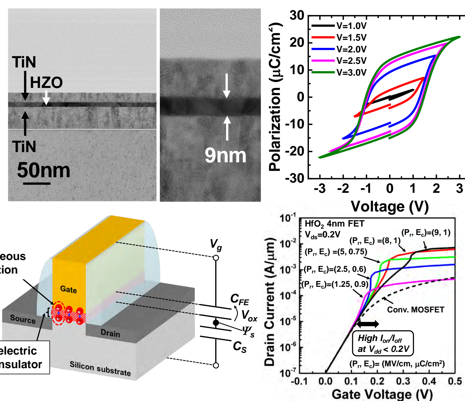
Fig. 3. (上) CMOS 集積化技術との整合性が高く次世代のロジック・メモリへの応用が期待される強誘電体ナノ薄膜技術。
