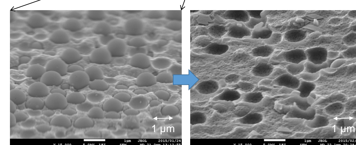
複合めっきを利用したロール金型表面とその転写結果
