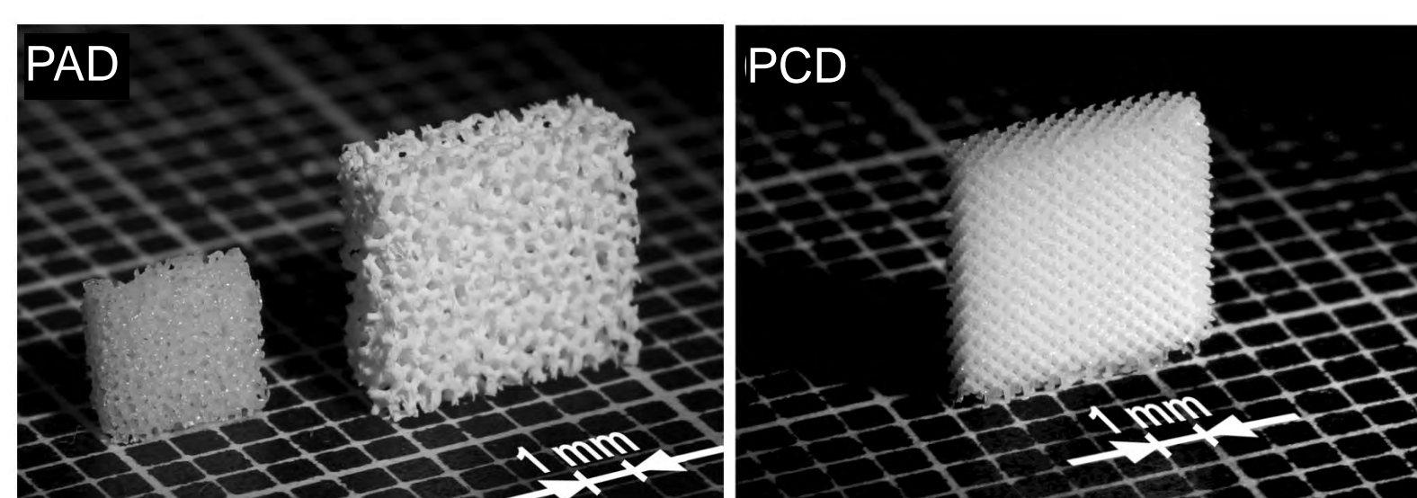
光禁制帯を形成することが期待される構造モデル(上段)およびテラヘルツ帯に光禁制帯を形成するように作製された誘電体の試料(下段)。それぞれ、アモルファス構造(左)および結晶構造(右)。
