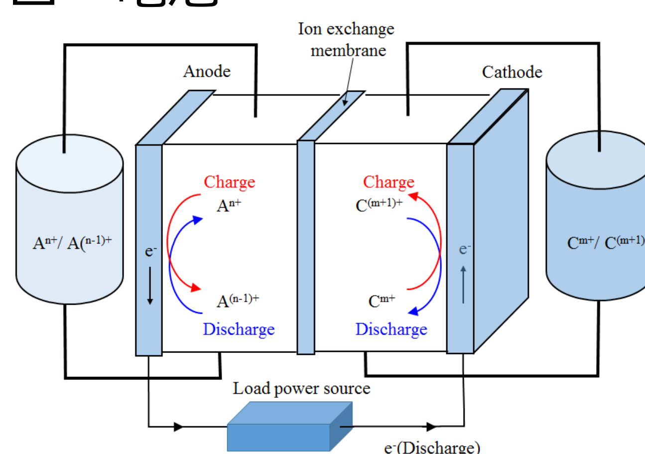
レドックス・フロー電池の模式図
