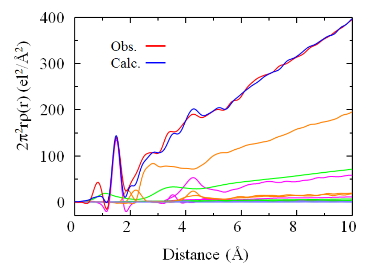
実測と計算による全相関関数
