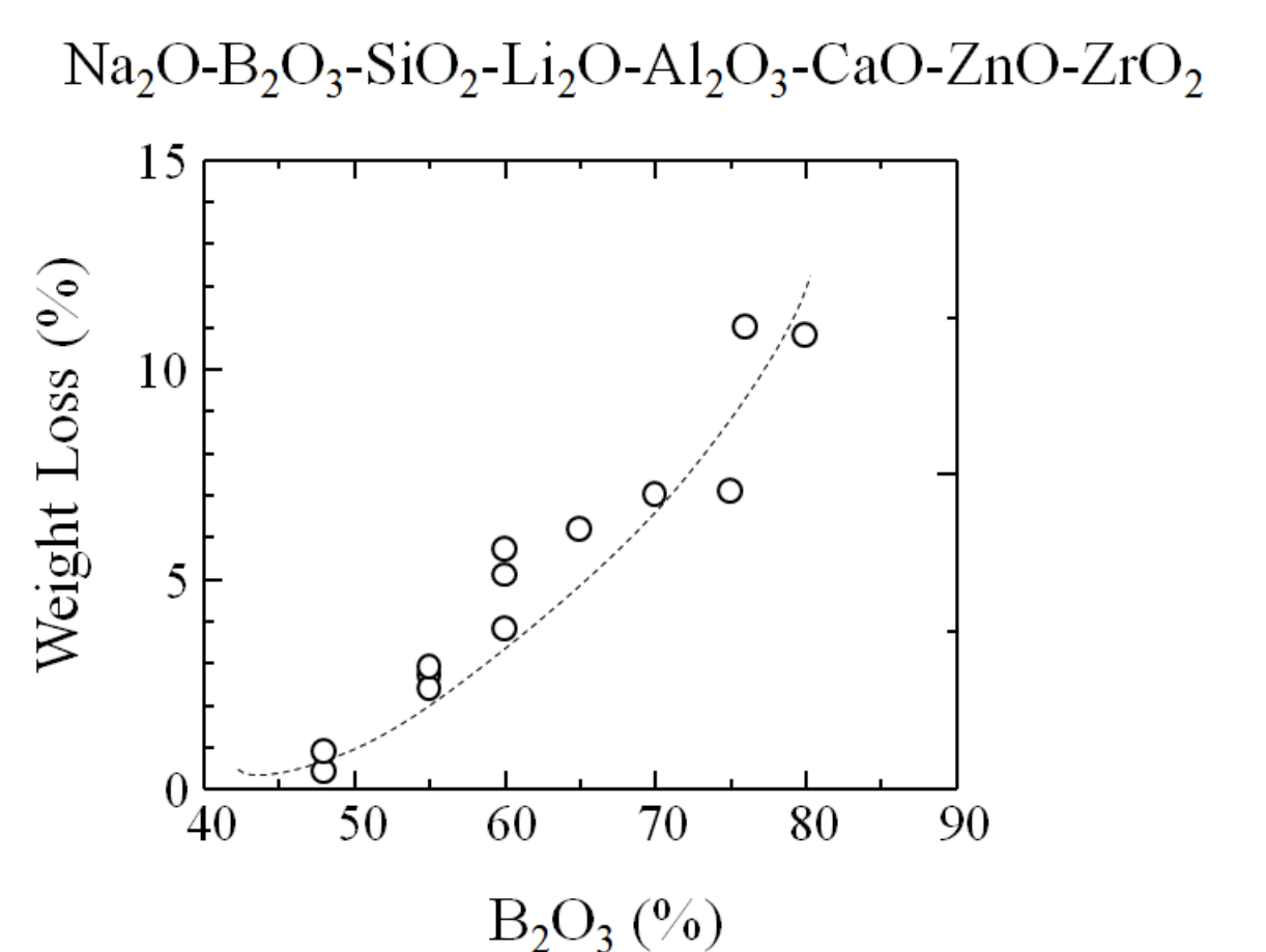
8成分系ガラスの分相処理後、熱水への溶出による重量減少率
