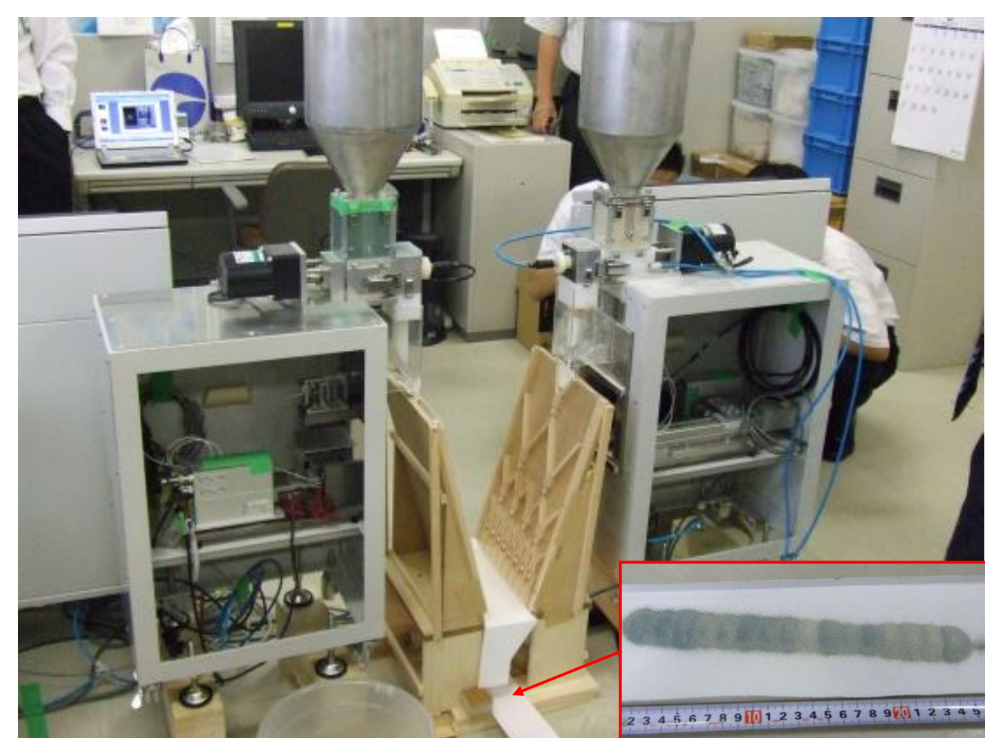
粉体の立体混合装置と、それを用いた Al 2 O 3 とSiCの混合物
