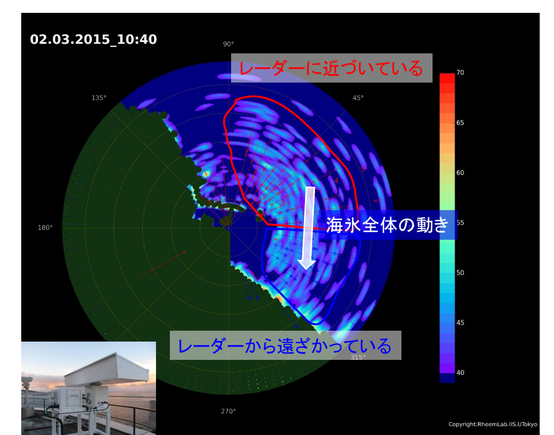
海氷観測レーダの観測結果
