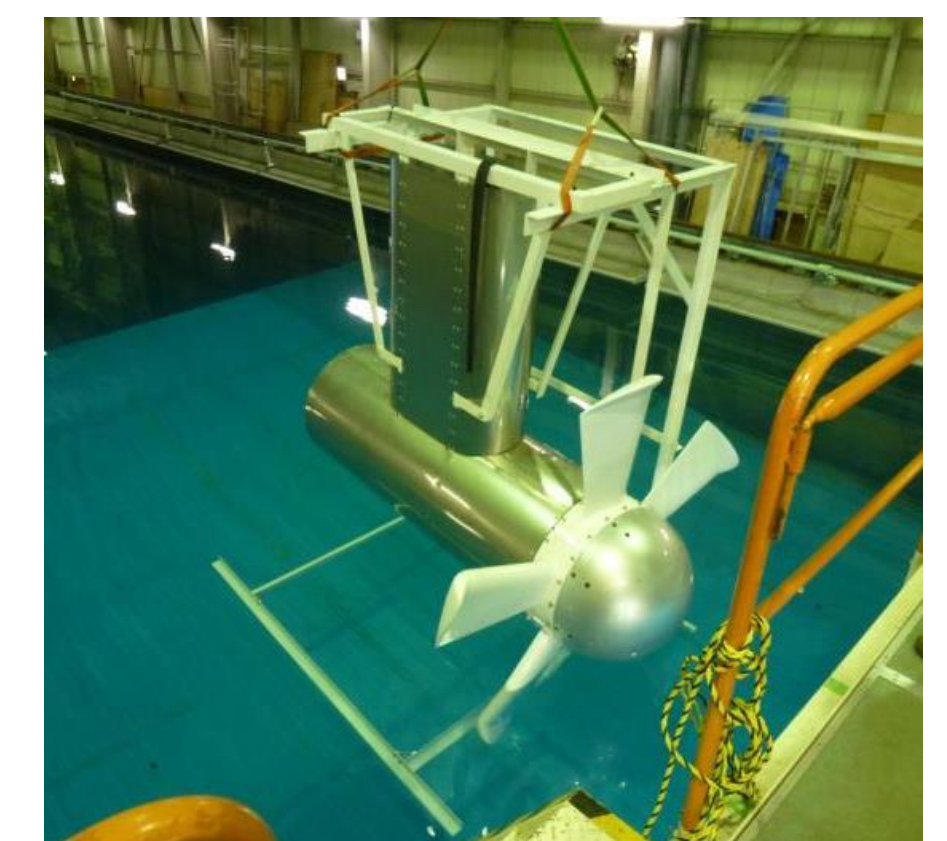
水槽における水車の性能試験
