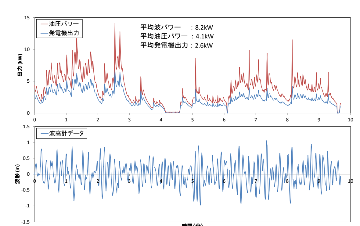
波力発電試験結果の例
