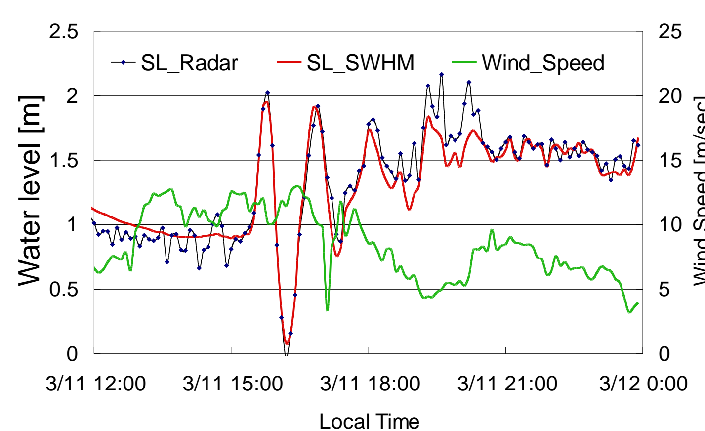
2011年3月11日相模湾で計測した津波
