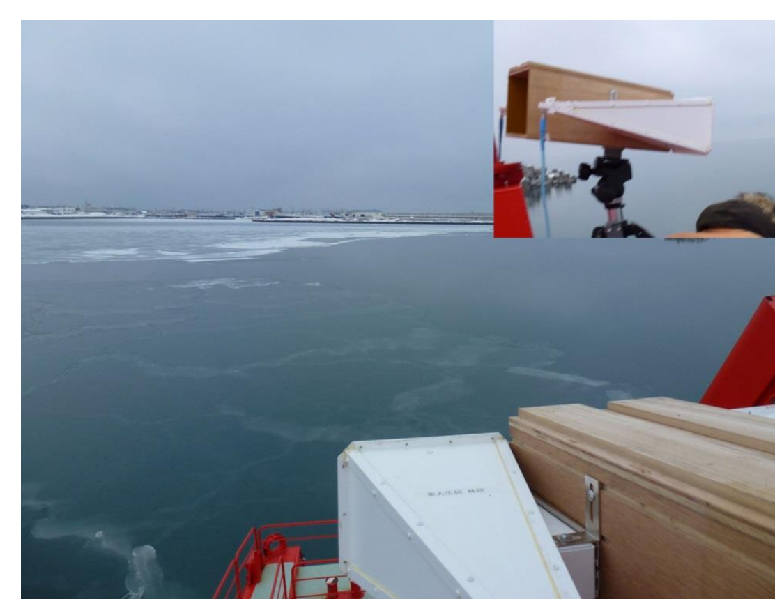
砕氷船におけるマイクロ波散乱実験
