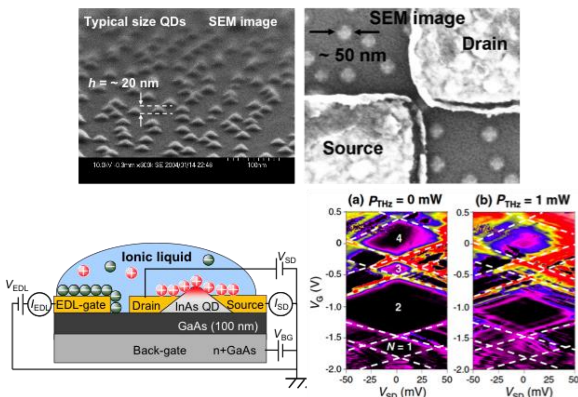
単一InAs量子ドットトランジスタの物理と応用
