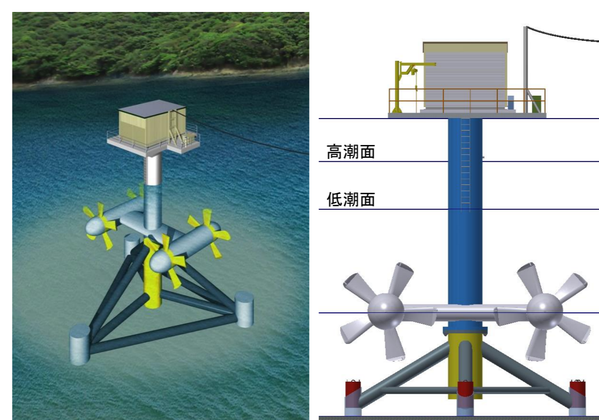
100kW 潮流発電装置
