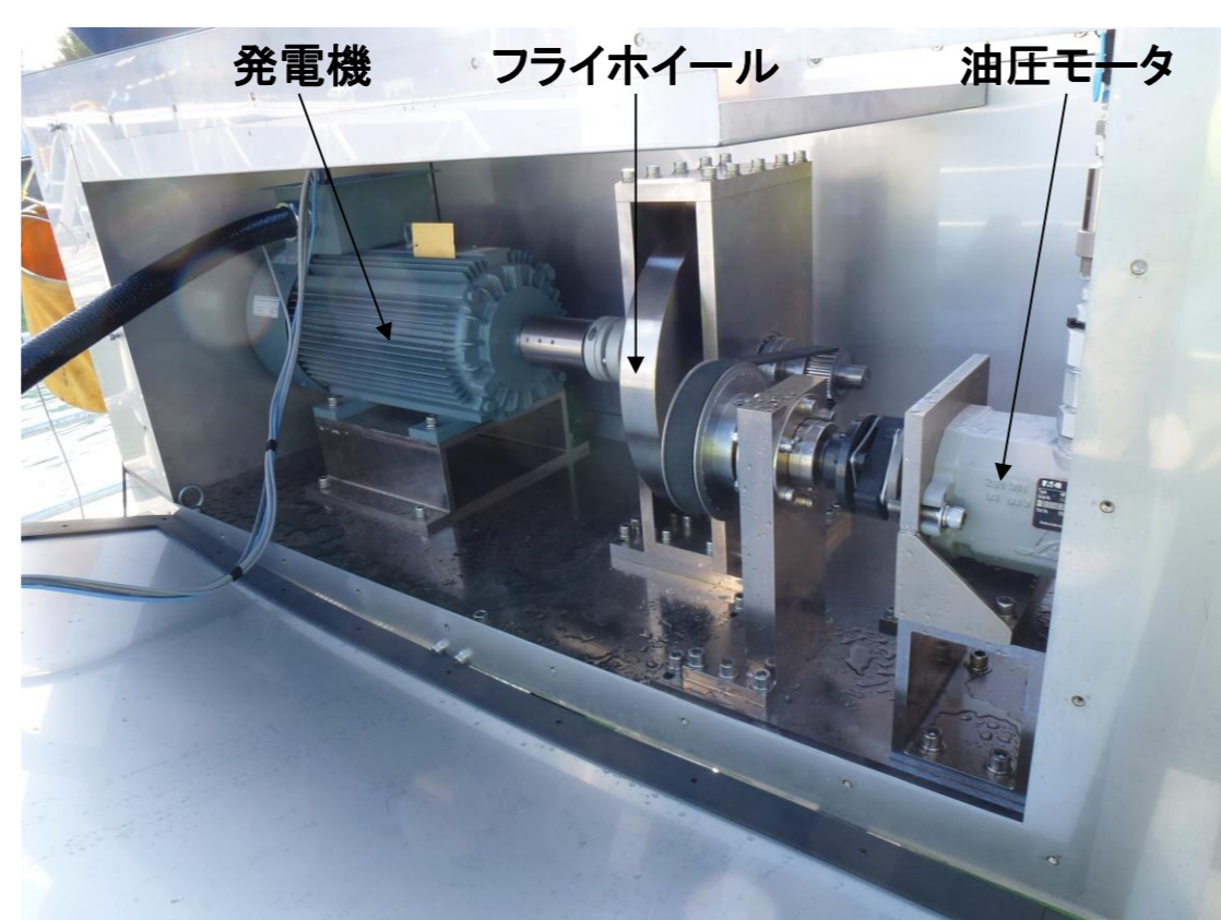
油圧発電システム
