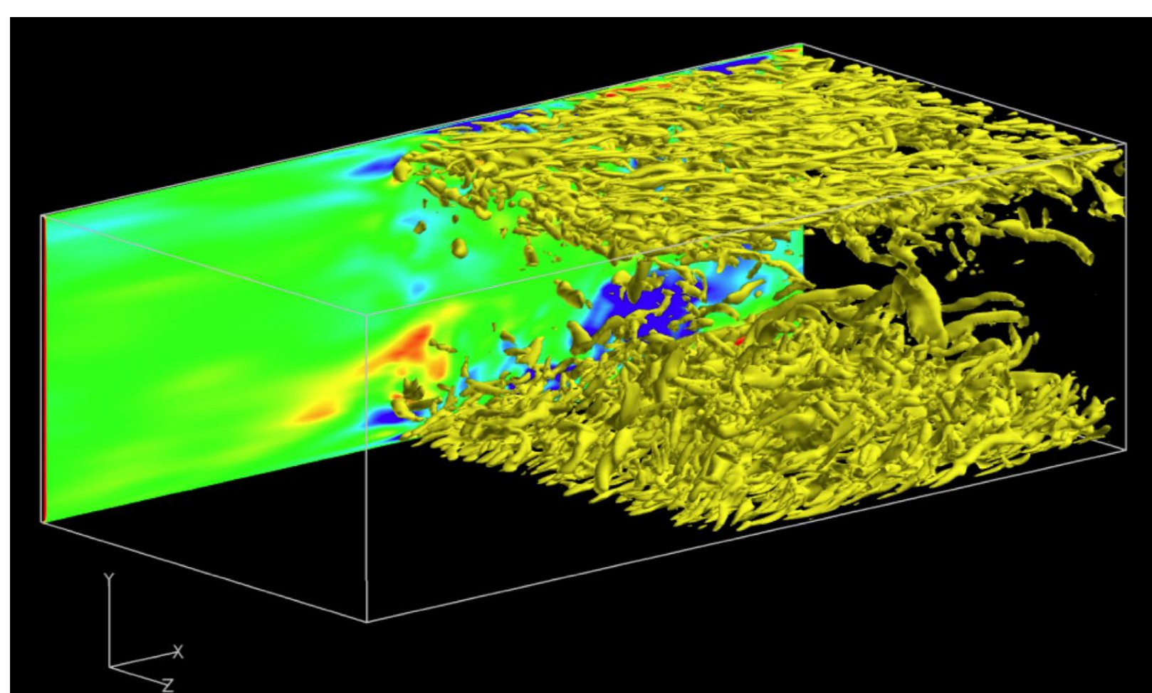
図1 チャンネル乱流の壁近くの渦
