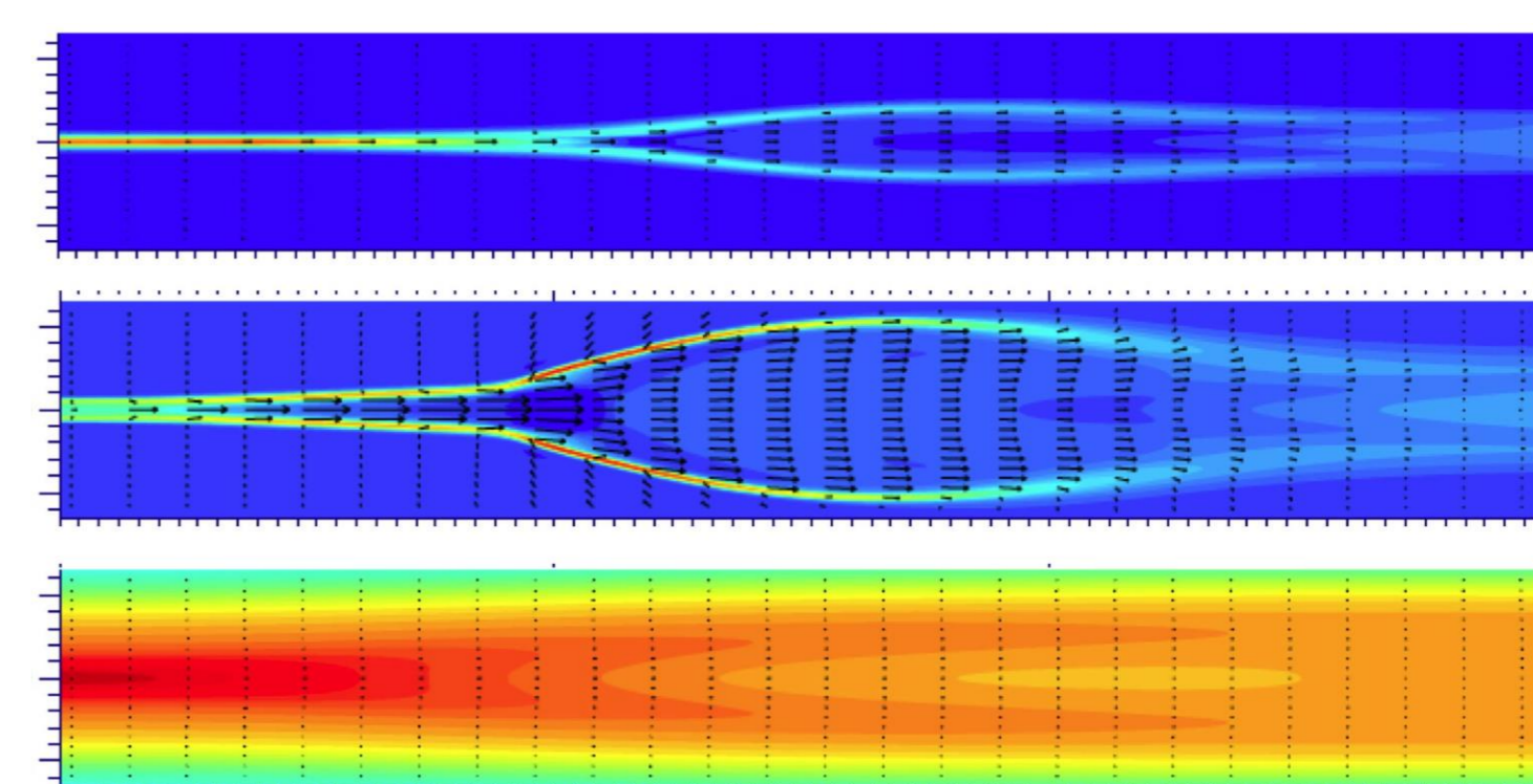
図3 磁気リコネクションのジェットと電流
