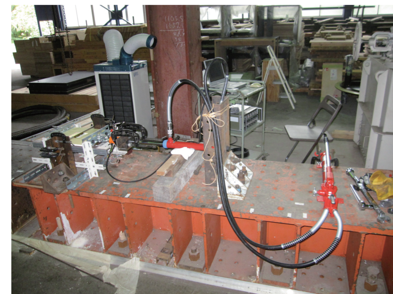
天井制振補強用金具の載荷実験
