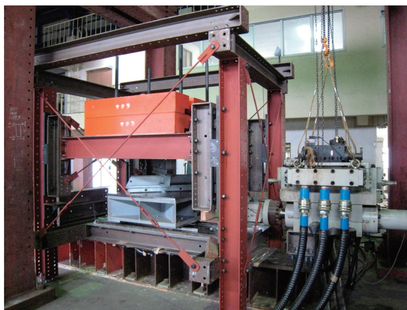
免震装置の性能試験
