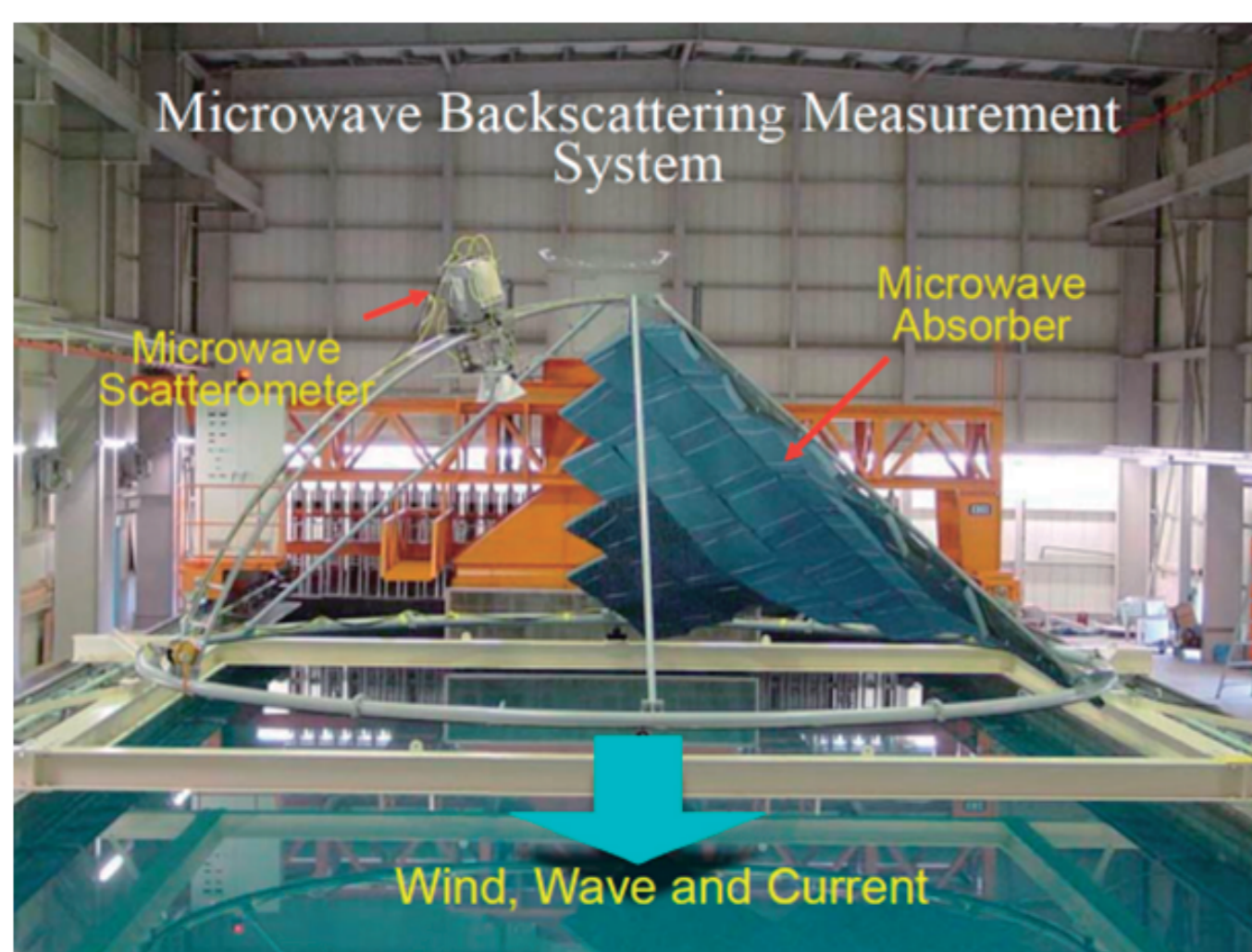
マイクロ波散乱の水槽実験
