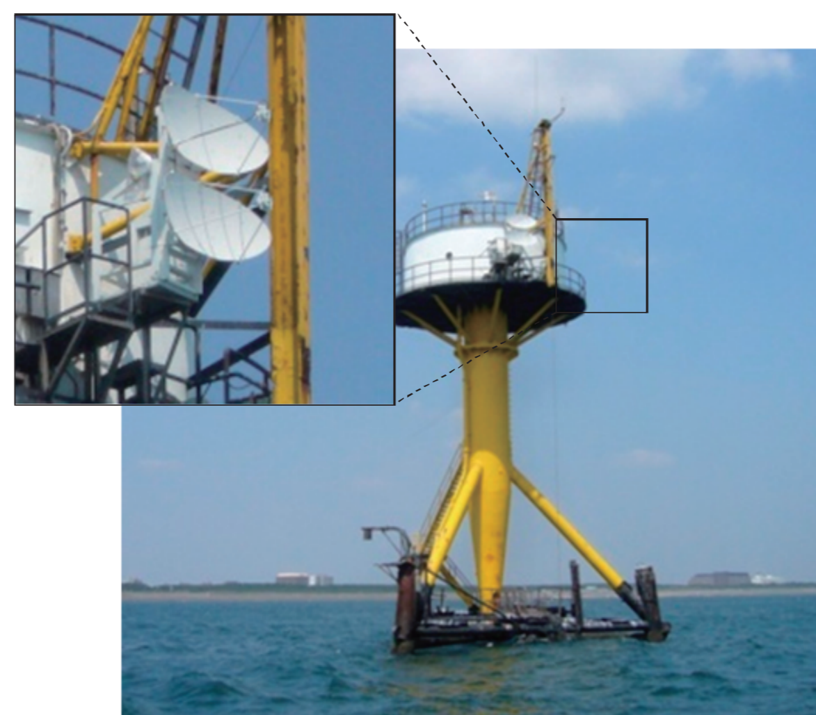
平塚沖総合実験タワーとマイクロ波レーダ
