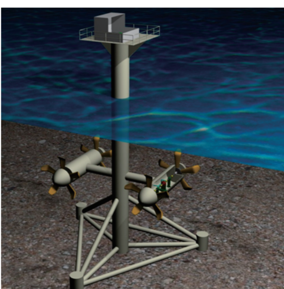
固定ヨー・ピッチ式潮流発電システム(100kW・250kW)
