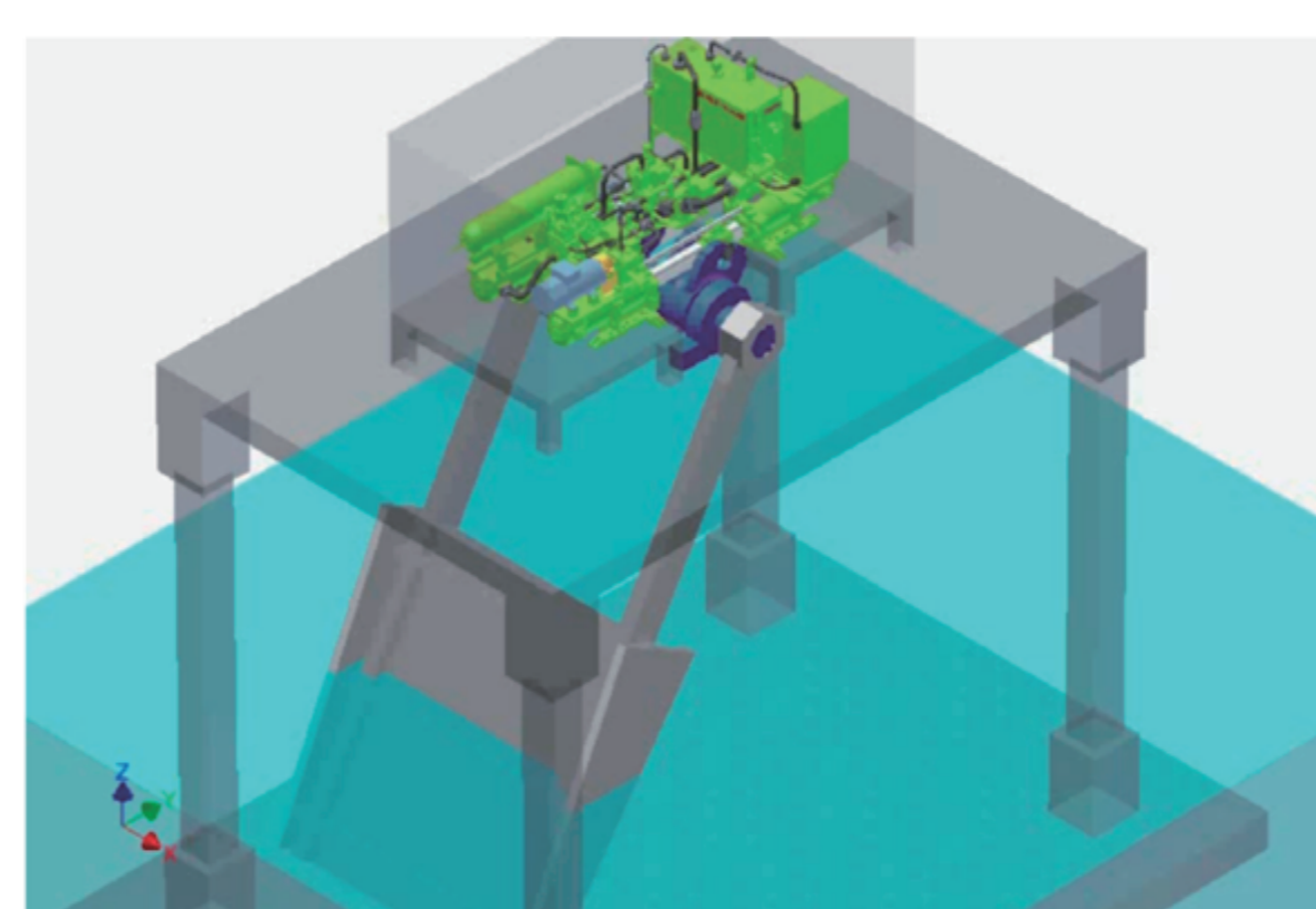
40kW 波力発電システム(岩手県久慈市)
