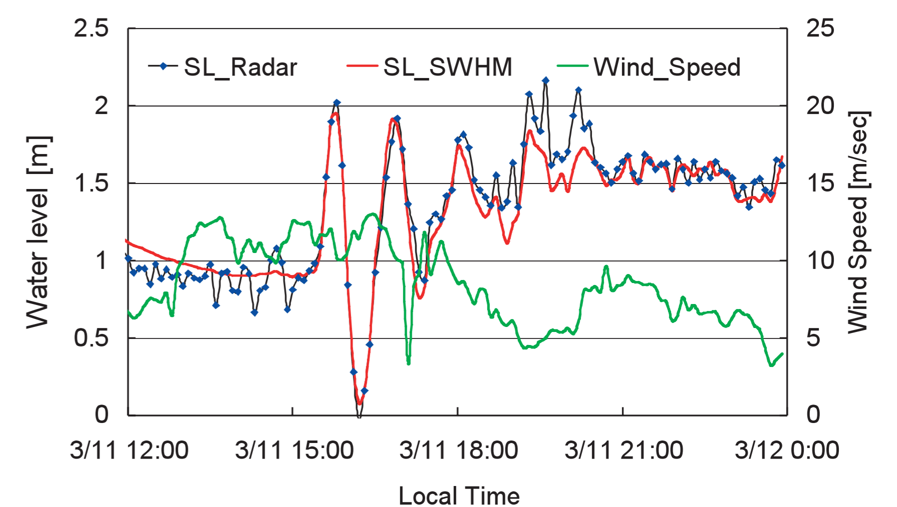
2011年3月11日相模湾で計測した津波
