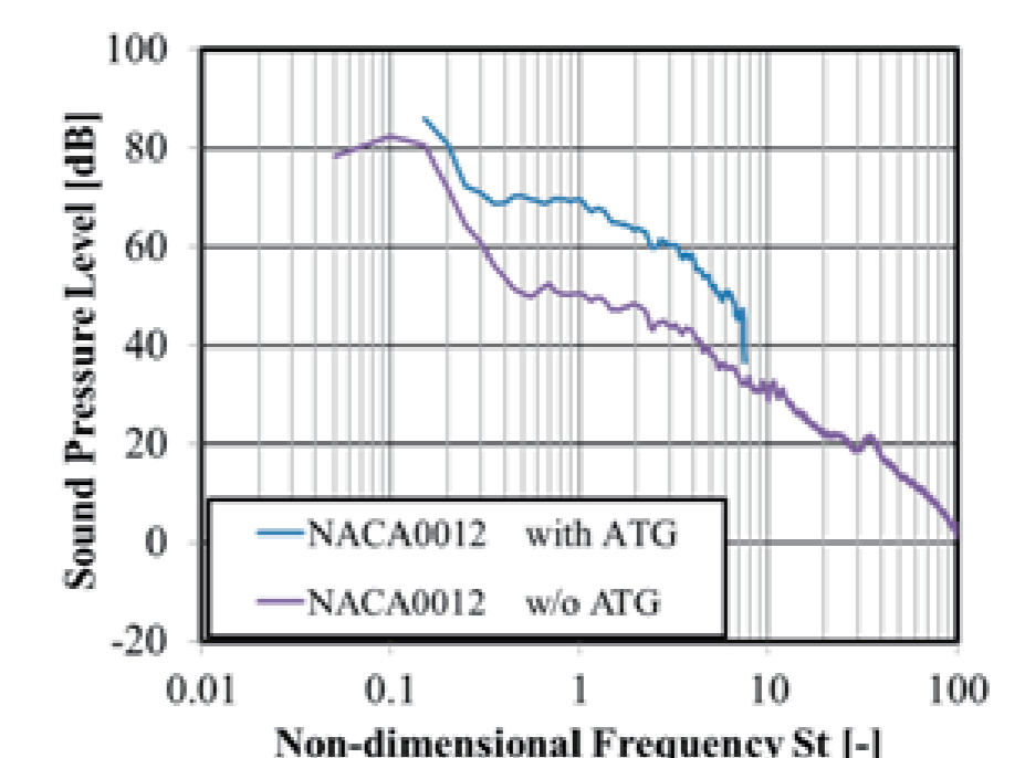
翼から発生するガストノイズの予測
