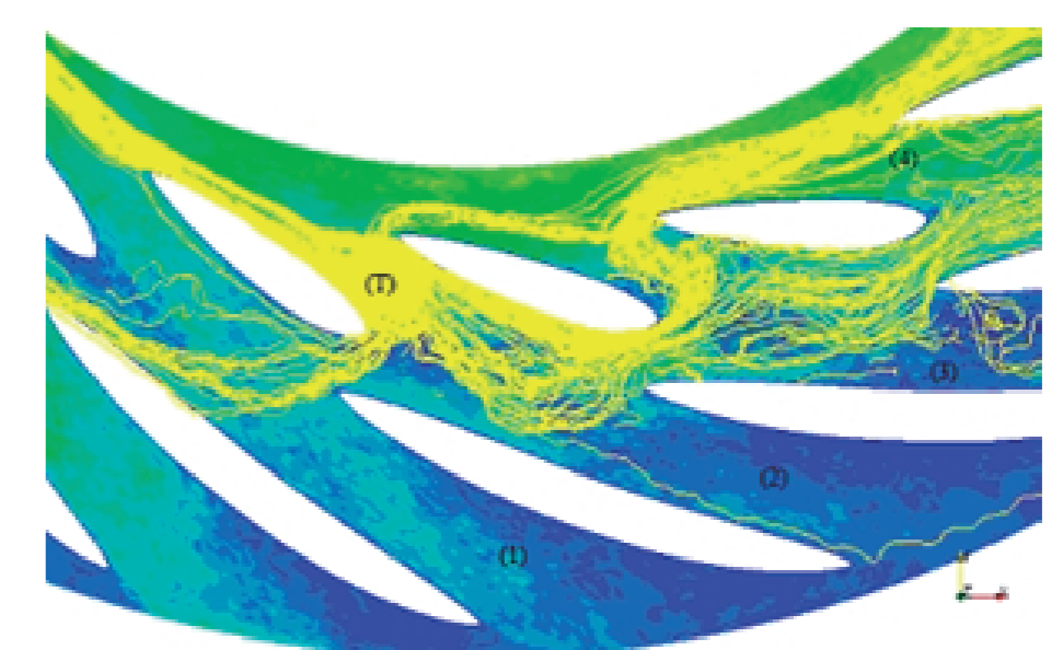
ポンプ水車内の旋回失速状態の解析
