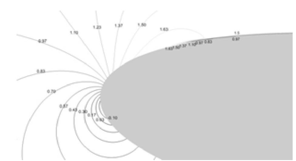
NACA0015翼まわりのキャビテーション解析
