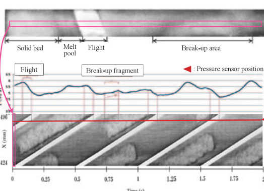
圧縮部におけるガラス短繊維強化PPの可塑化過程
