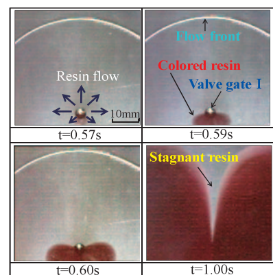
ホットランナー金型における樹脂色切替時のキャビティ内充填挙動
