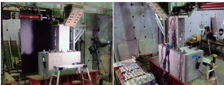
(a) 試験体 (FS-90試験体) 正面 (b) 試験体 (FS-90試験体) 背面 静的載荷実験の様子
