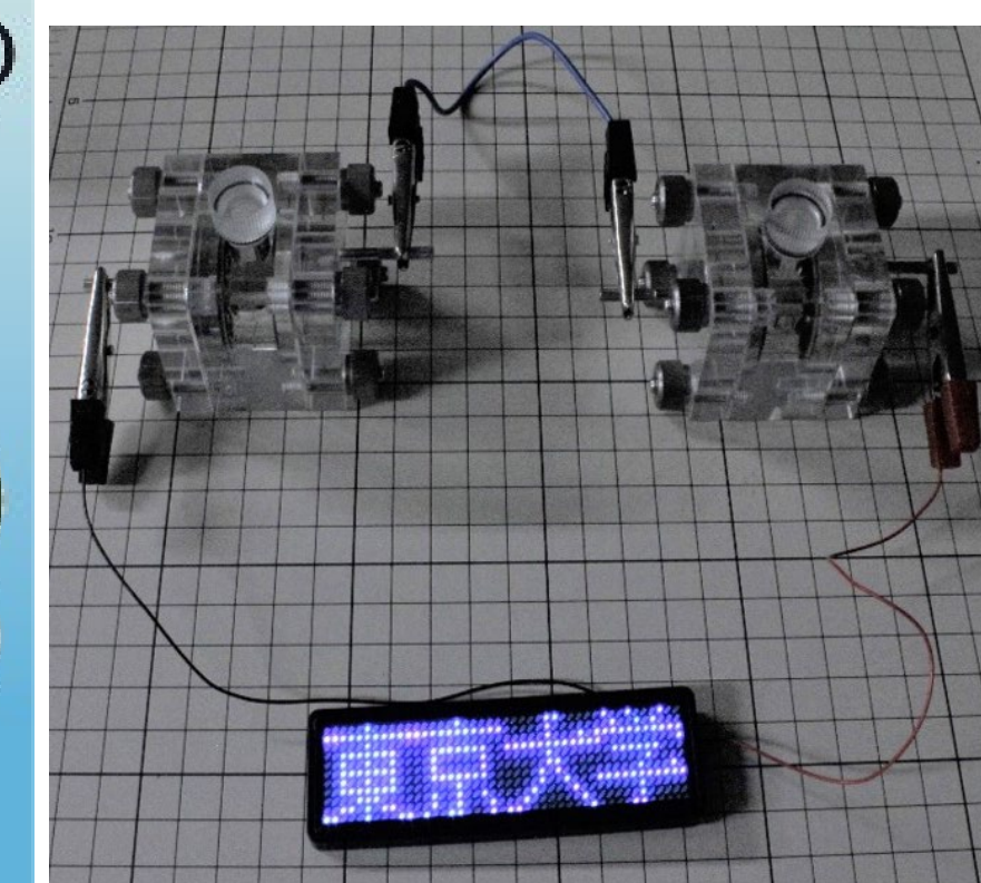
試作した金属空気電池
