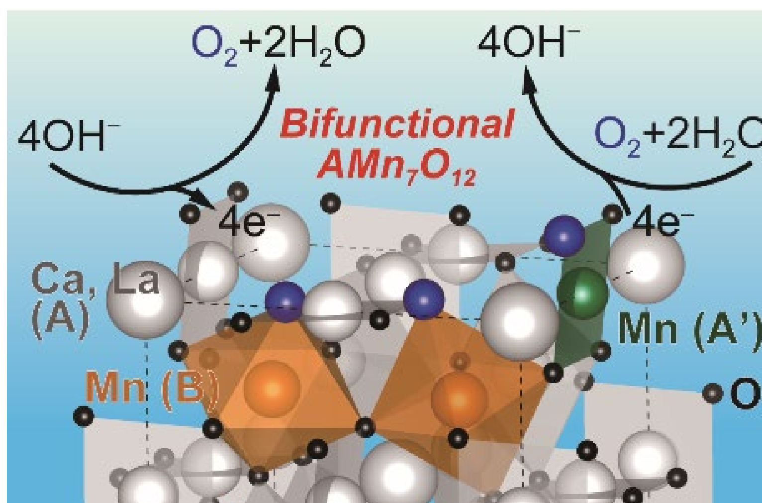
酸素発生反応と酸素還元反応の両方に活性を有する二機能性触媒CaMn 7 O 12
