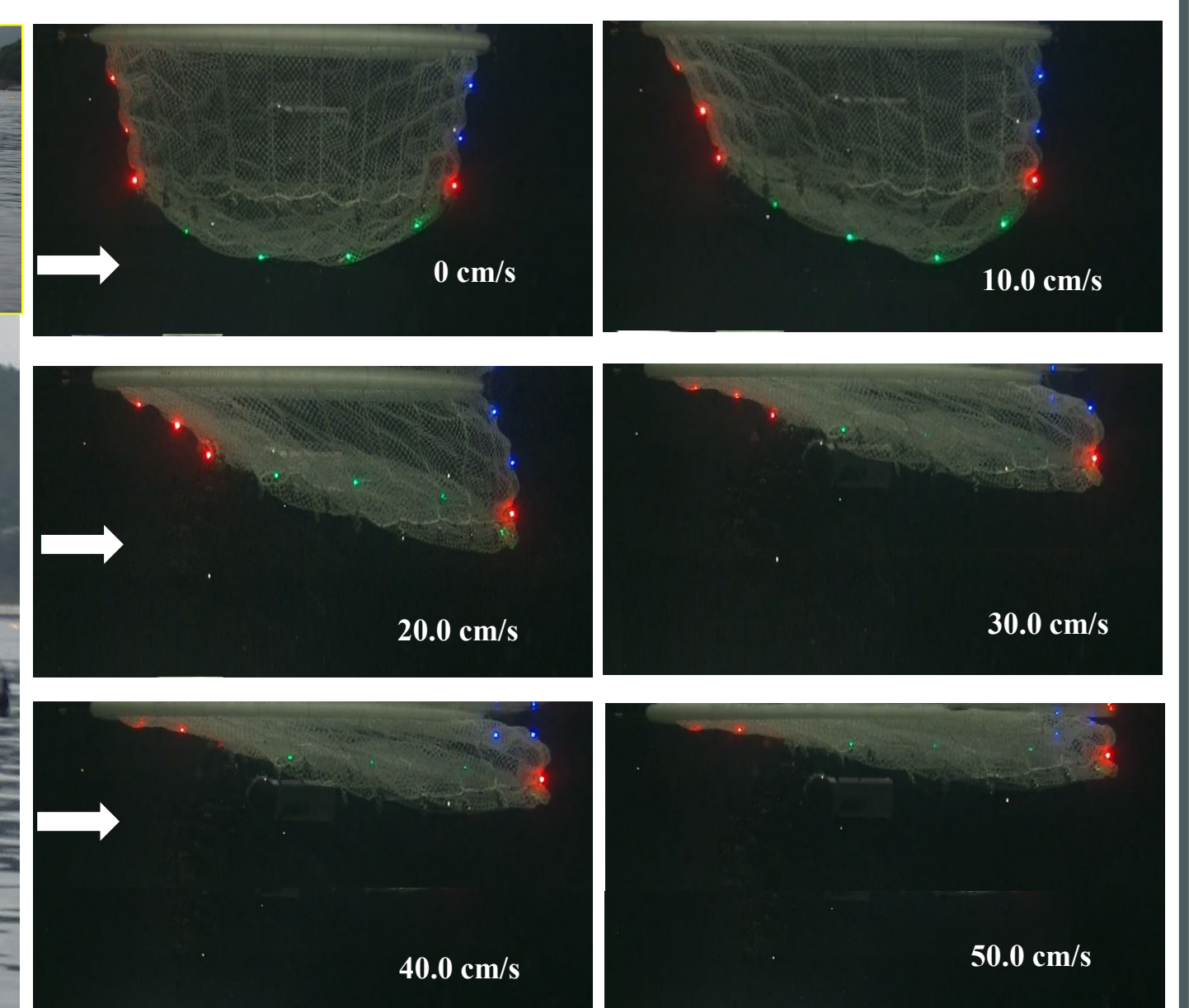
柔軟な網生簀構造物の変形 流速が大きくなると網地が大きく変形します。
