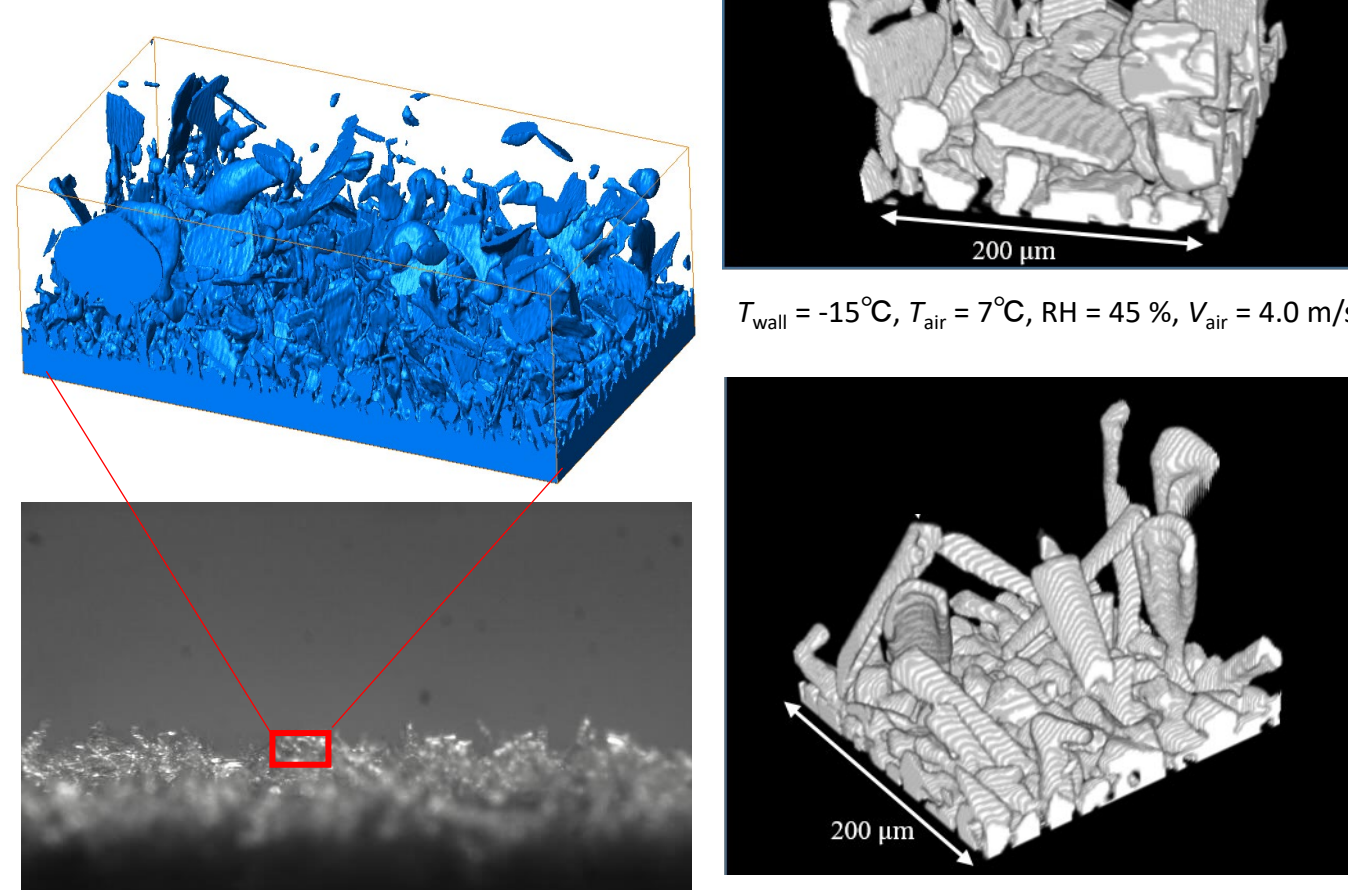
霜構造の3次元計測
