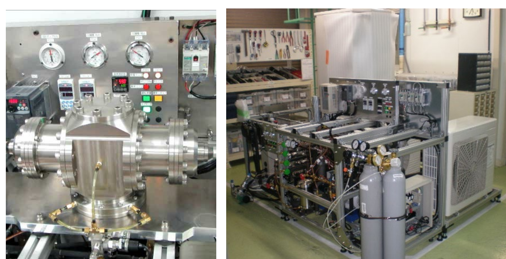
トリラテラルサイクル用膨張機および実証装置
