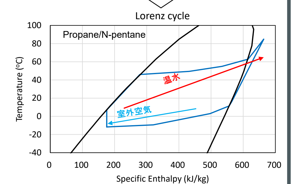
大温度グライドで高効率なローレンツサイクルヒートポンプ
