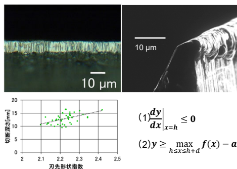
研磨した刃物先端の形状と切れ味の関係
