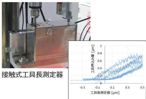
工具接触検知の繰り返し試験
