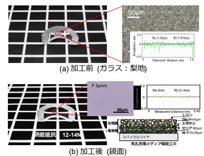
超長寿命・微粒固定砥粒工具による粗面ガラスの鏡面化
