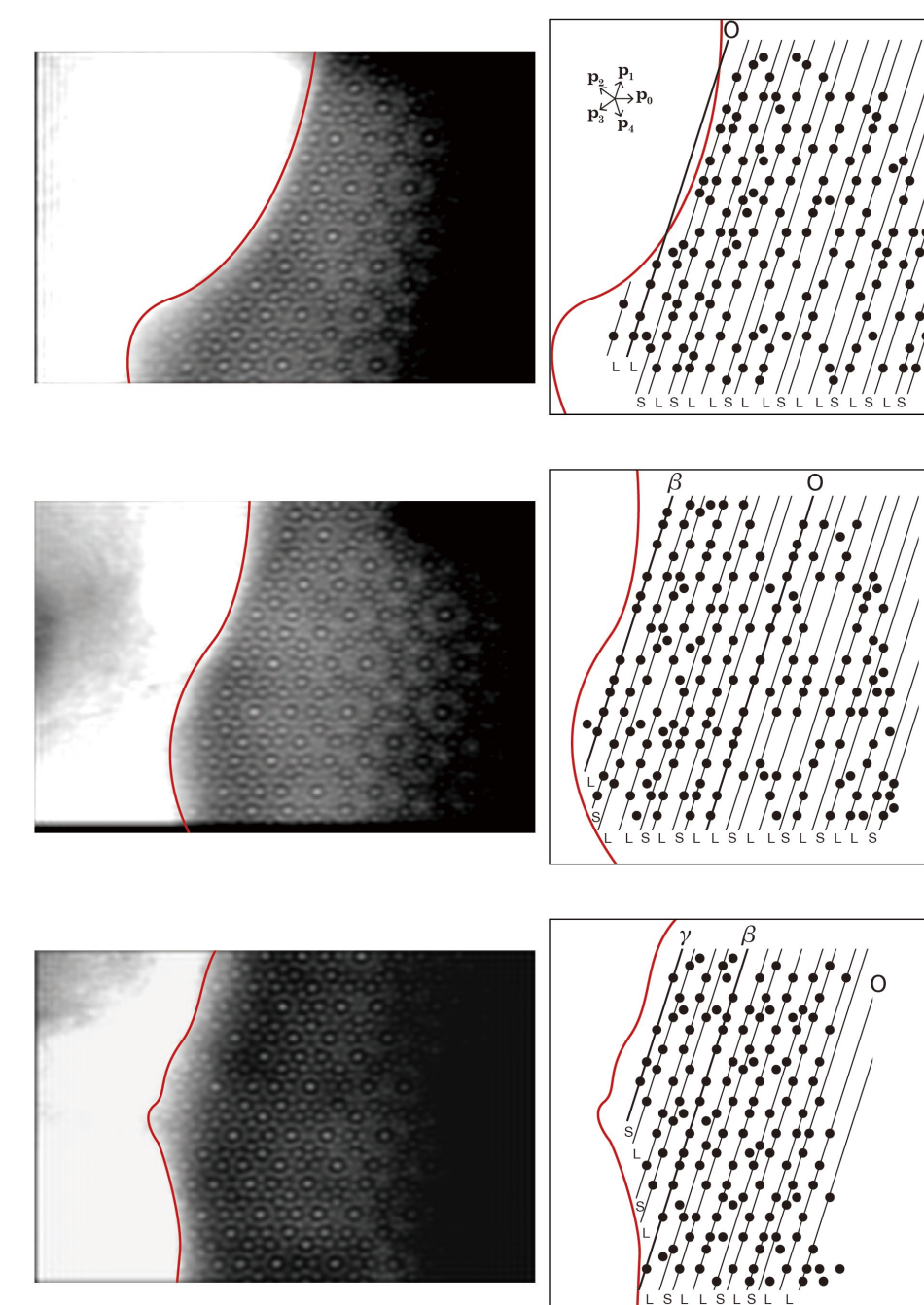
Al-Ni-Co系正10角形準結晶の成長の様子の透過電子顕微鏡高温その場観察
