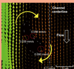
赤血球膜の回転運動と赤血球周りの流速分布
