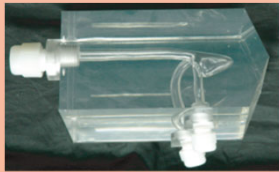
脳動脈瘤の実血管形状モデル
