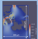
血流シミュレーション結果を用いた薬剤ミセルのトラップ位置の解析
