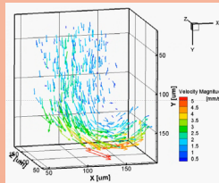
液滴内の3次元流動
