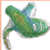
動脈瘤内の流線
