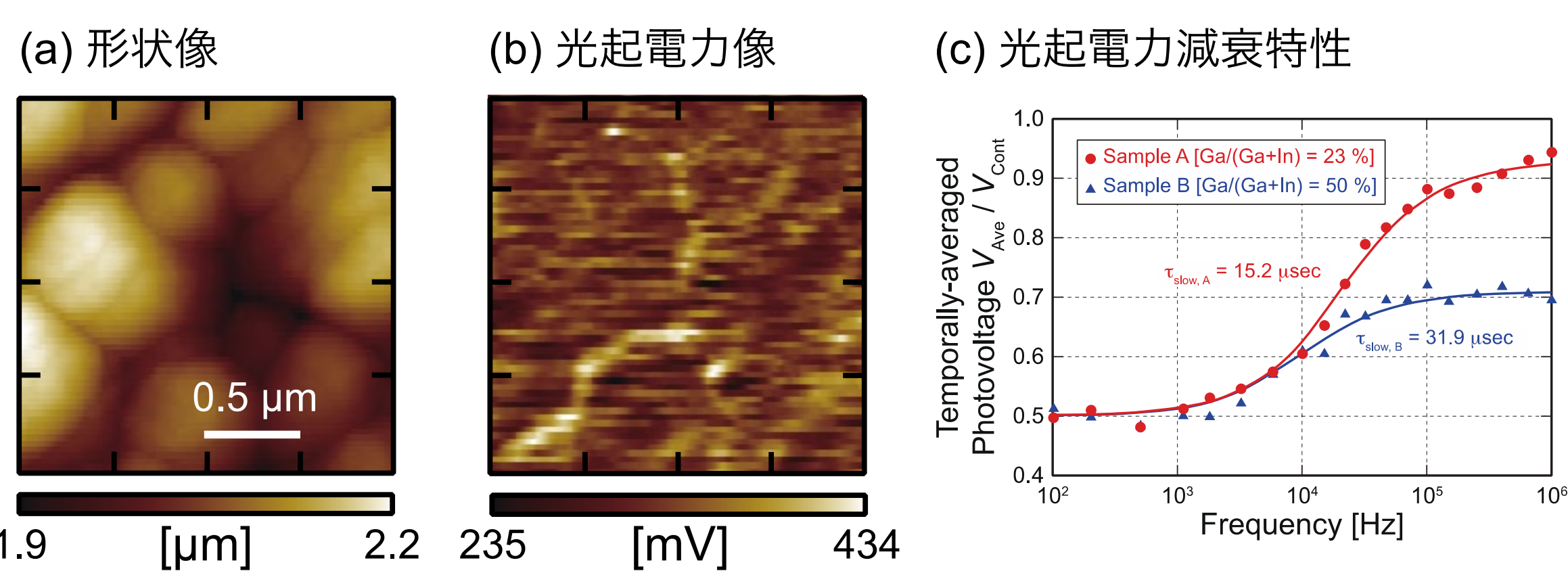
CIGS太陽電池における形状像と光起電力像、および、光起電力減衰特性
