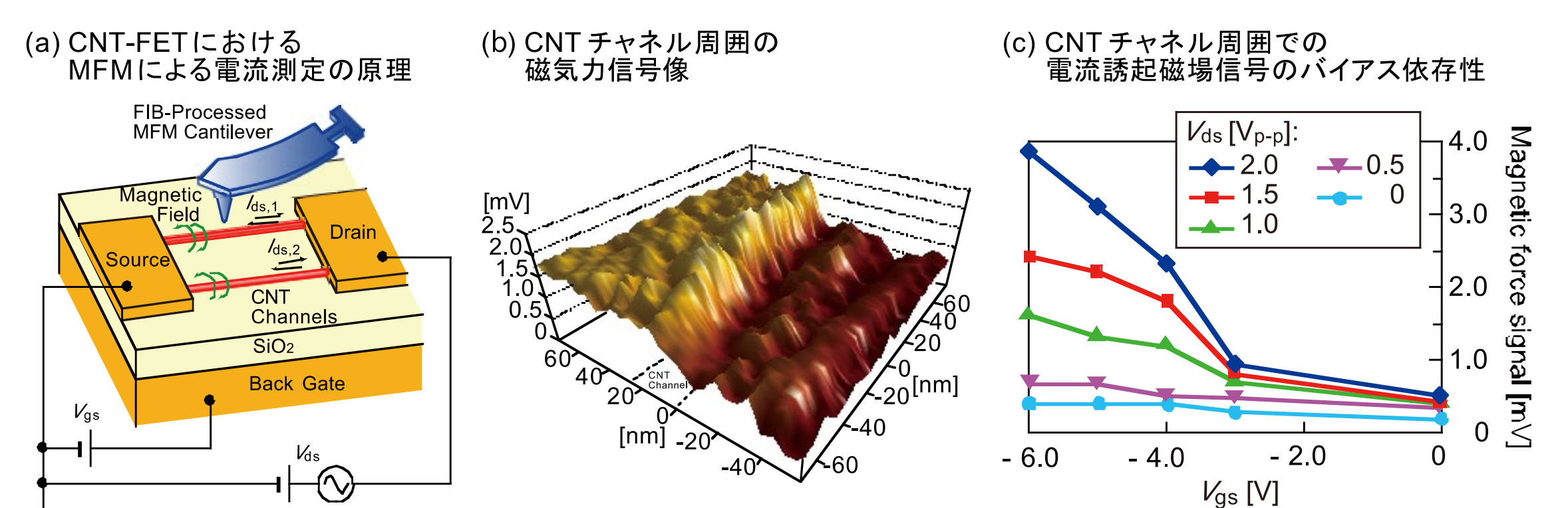
MFM電流誘起磁場計測系によるカーボンナノチューブFETチャンネルの評価
