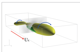
図1 チャネル乱流の壁近くの渦構造
