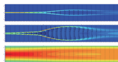
図3 磁気リコネクションのジェット
