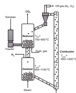
CO 2 フリー水素製造システム
