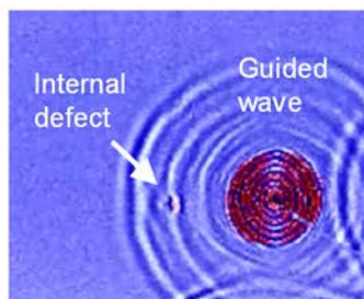
超音波伝播挙動の可視化
