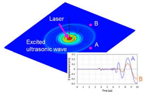
レーザー超音波の数値シミュレーション
