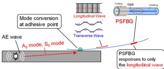
高温環境でのAE計測が可能な遠隔センシング法
