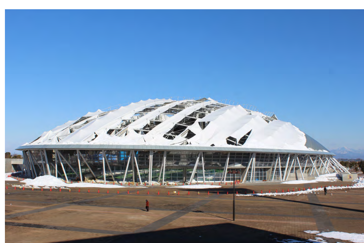
2014年2月14日の大雪による屋根崩落被害の調査
