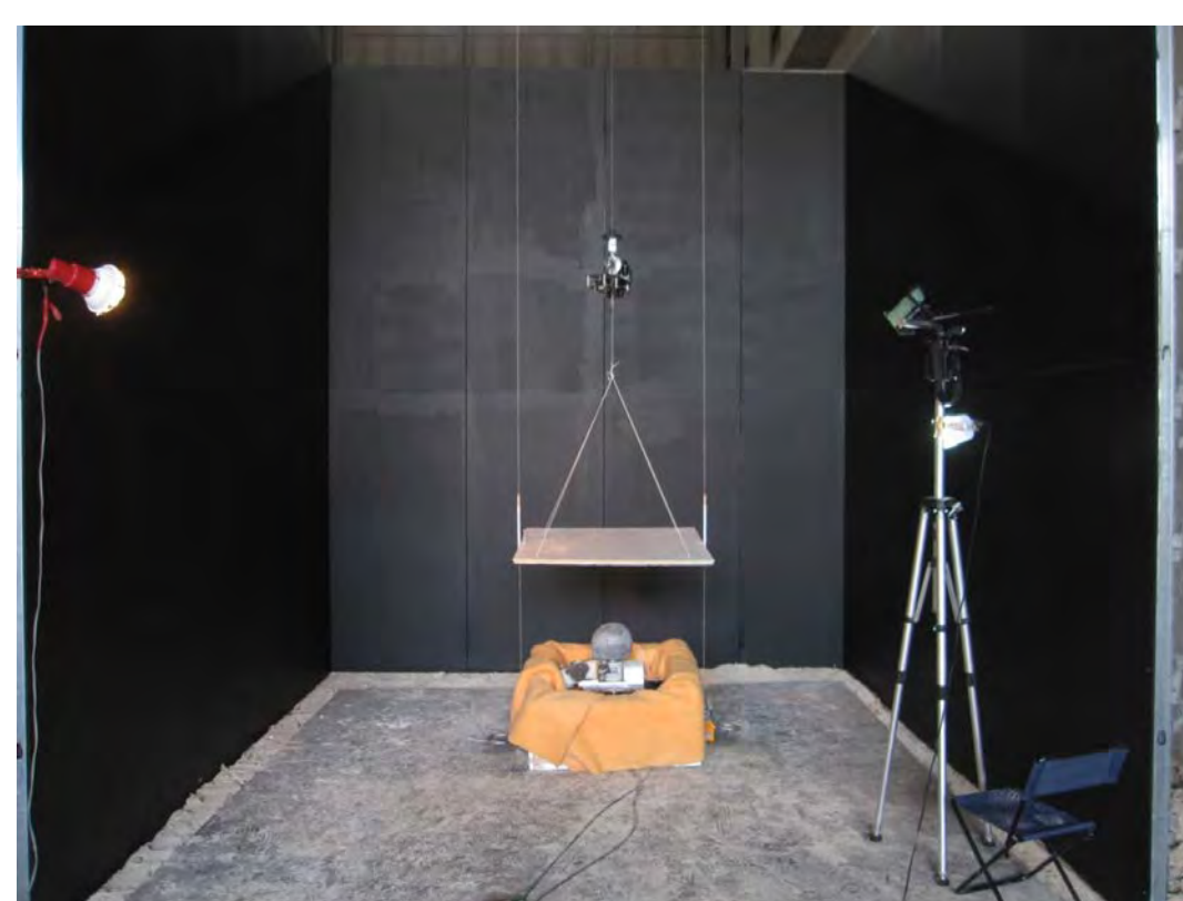
天井材落下実験による安全性評価
