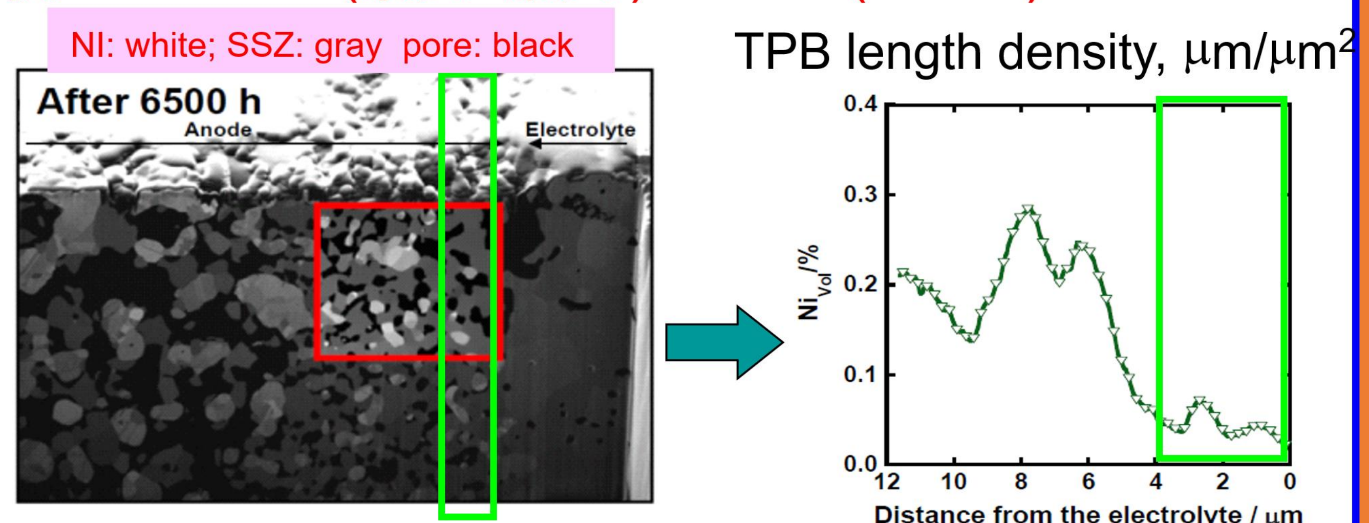
図1. TOTO製円筒縦縞形セルの劣化例（産総研のSIMS観測によって、P, Siが電気化学的活性点濃集していること、京大・東大のFIB・SEM分析によって、活性点からNiが後退していることが明らかになった）
