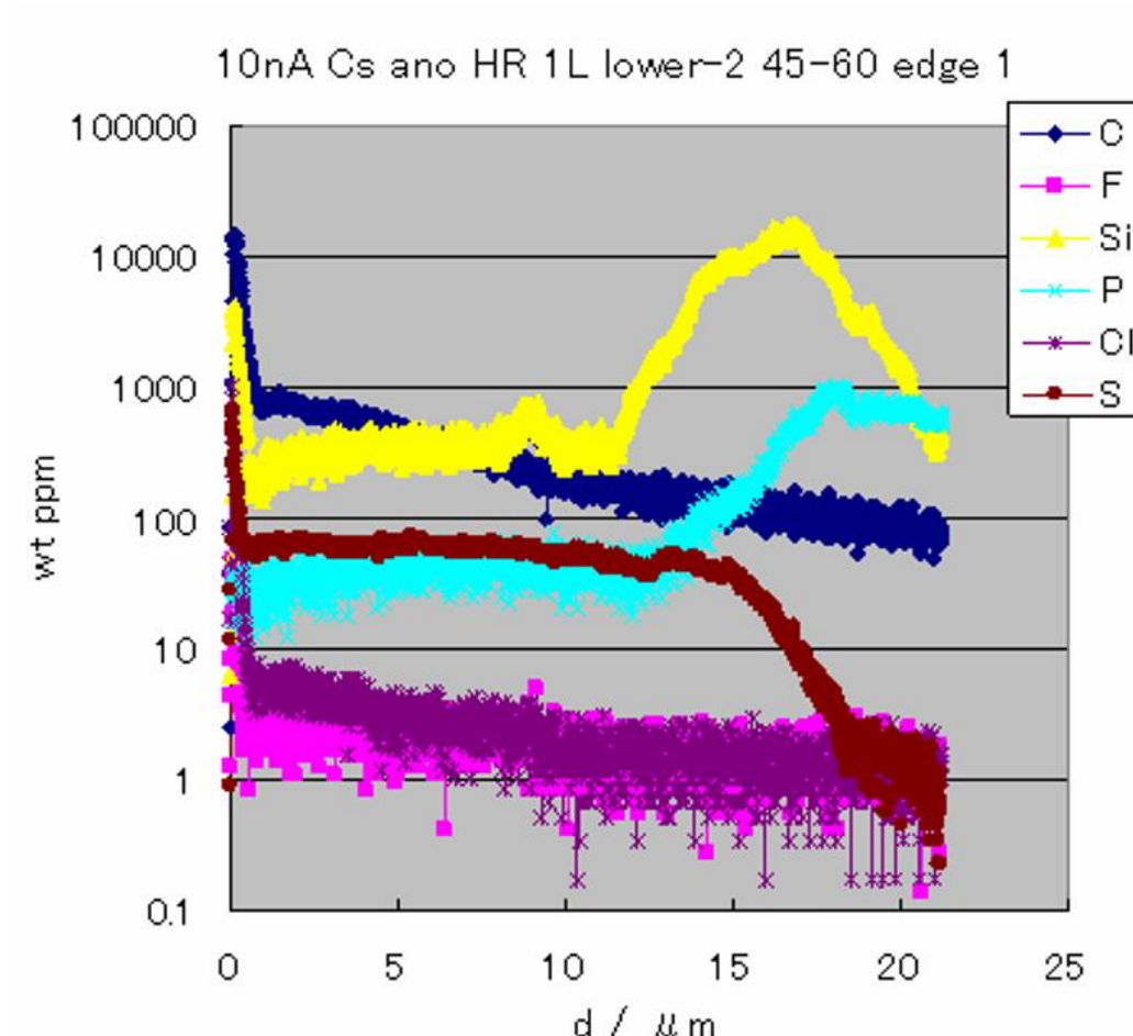
図1. TOTO製円筒縦縞形セルの劣化例（産総研のSIMS観測によって、P, Siが電気化学的活性点濃集していること、京大・東大のFIB・SEM分析によって、活性点からNiが後退していることが明らかになった）
