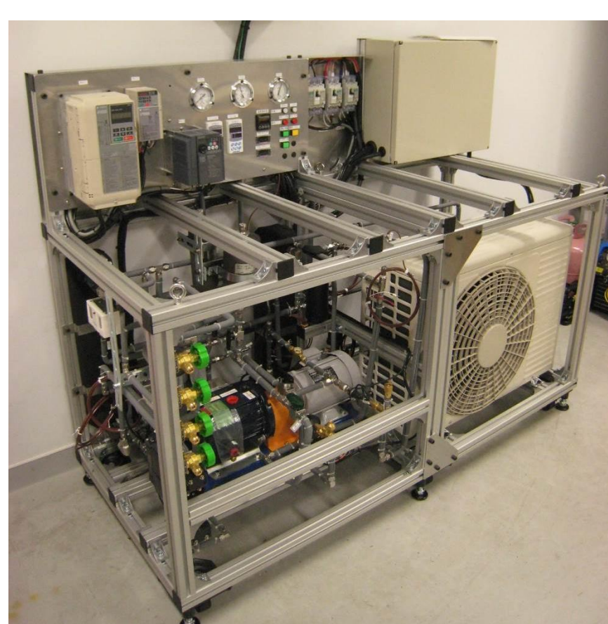
トリラテラルサイクル用膨張機および実証装置
