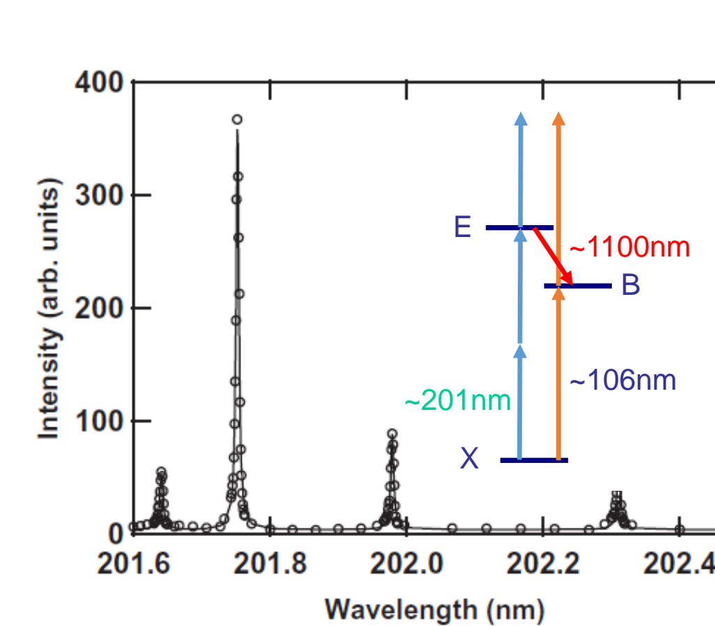
[水素の回転分光]
