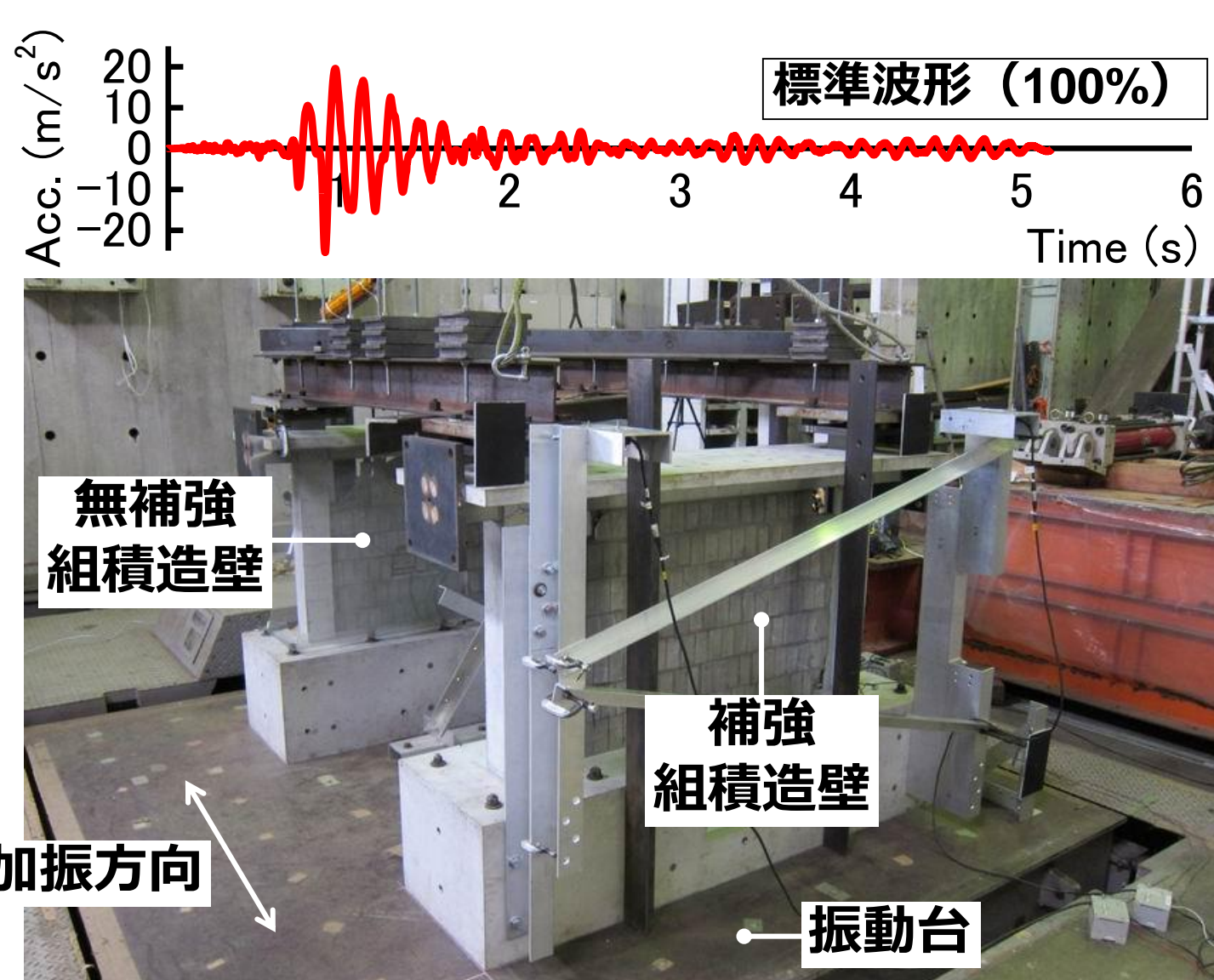
振動台実験の様子および入力標準加速度波形
