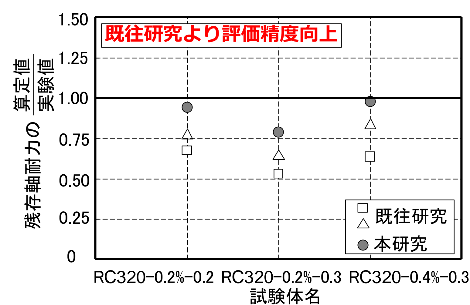
残存軸耐力の算定値と実験値の比率
