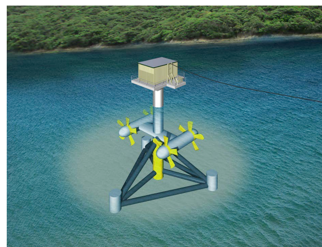
100kW 潮流発電装置
