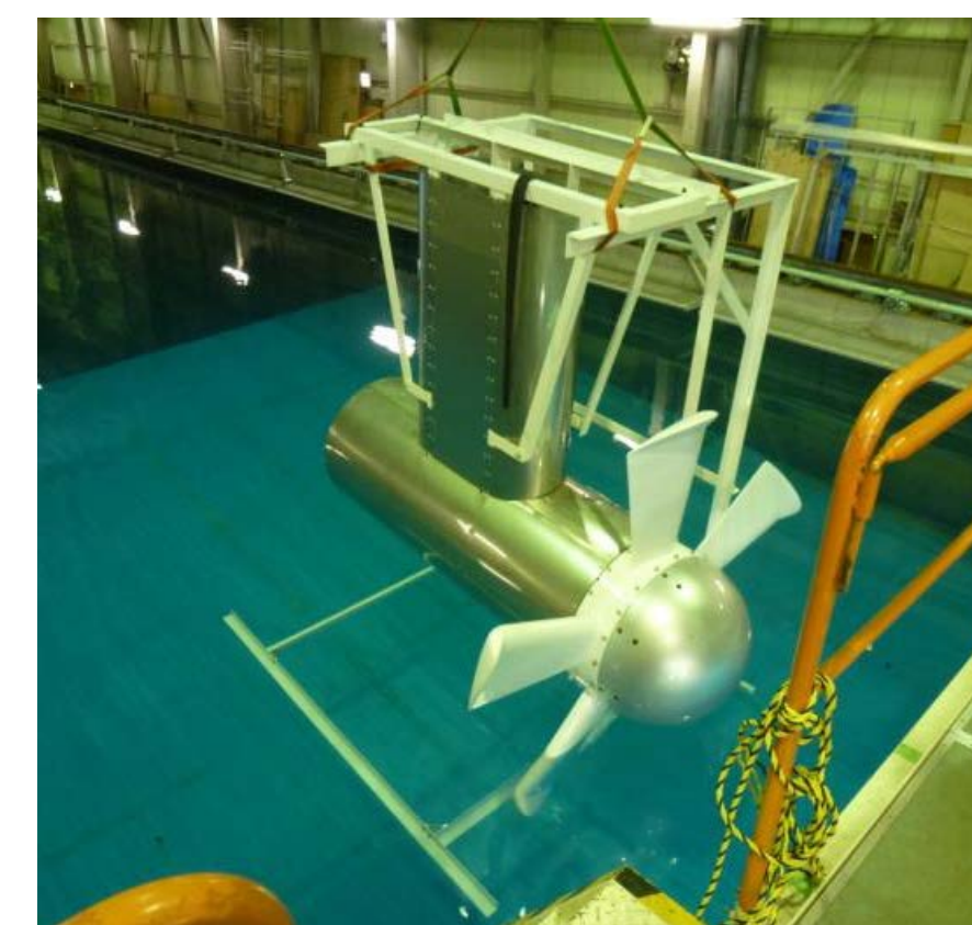
水槽における水車の性能試験
