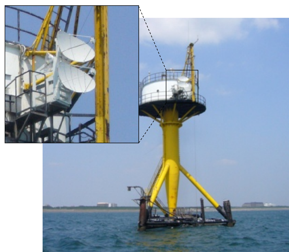
平塚沖総合実験タワーとマイクロ波ドップラーレーダ
