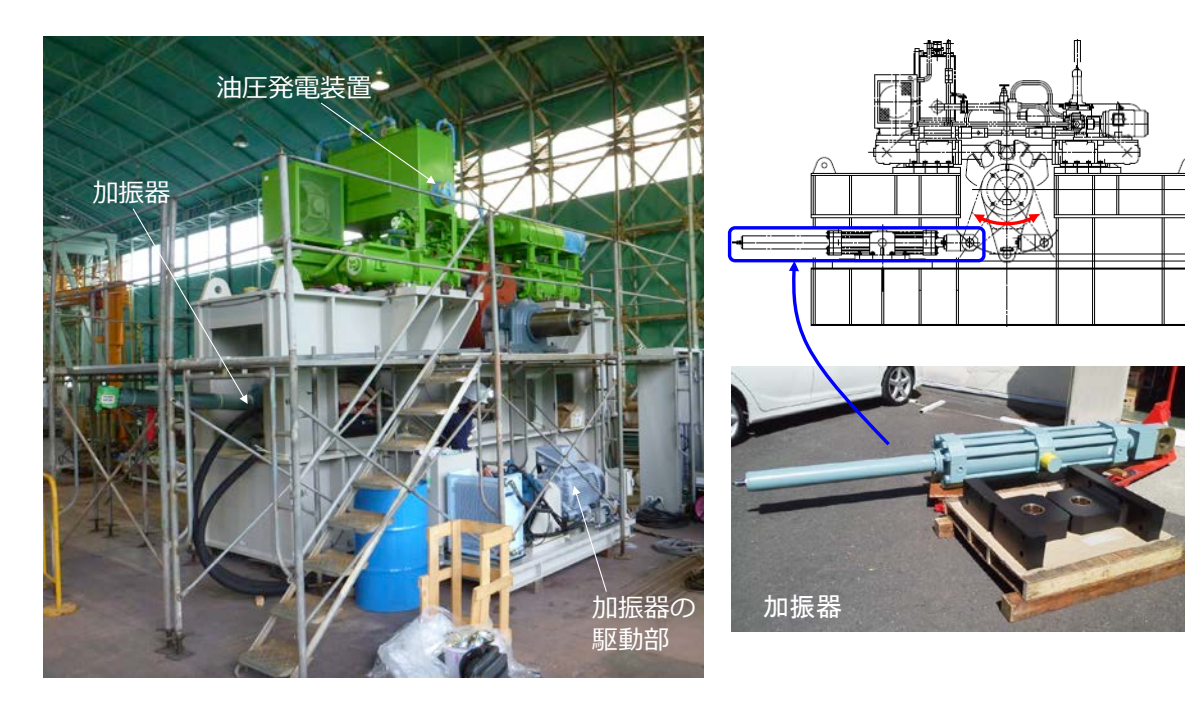
油圧発電装置の陸上ベンチ試験
