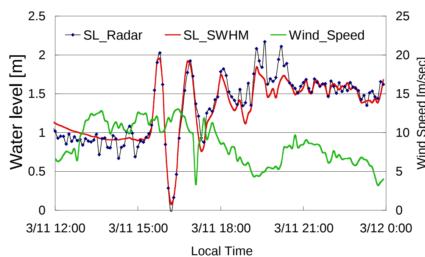
2011年3月11日相模湾で計測した津波
