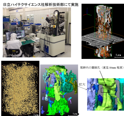
FIB-SEMIによるコンクリート中の空隙の観察と物質移動を支配する閾細孔径の検討
