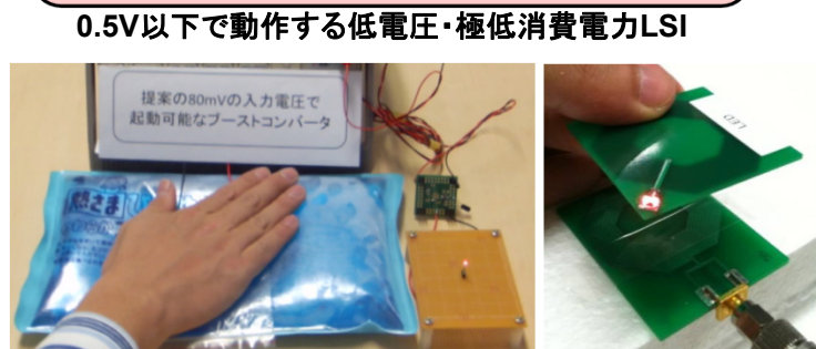
温度差発電(左)と無線給電(右)でLEDを点灯
