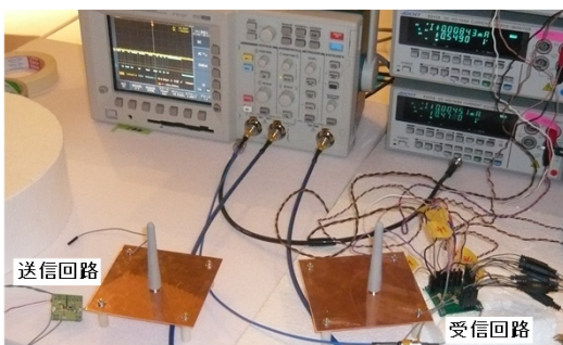
1Mbpsを100 \mu\text{W} 以下で実現した無線トランシーバ
