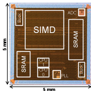
図2 0.6V動作320並列SIMDプロセッサのチップ写真(左)と動画画像フィルタ処理のデモ(右)
