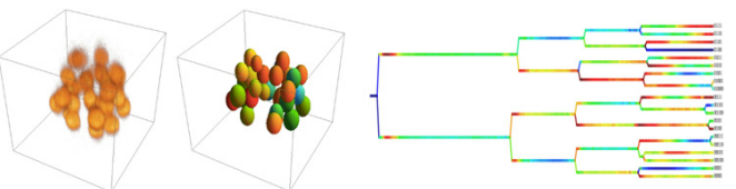
図1. 哺乳類発生の画像解析
