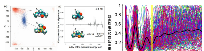
図3. ポテンシャルに基づく、ペプチド構造変化のPCA解析
