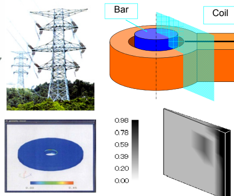
溶融亜鉛めっき中の脆化割れ、 高周波焼入れによる硬化層の生成 (電磁場・熱・力学・相変態)
