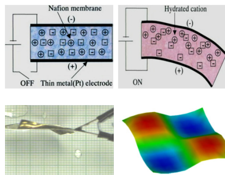
導電性高分子アクチュエータの電気化学・力学応答
