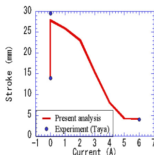
強磁性形状記憶合金アクチュエータの磁場・超弾性応答
