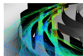
ポンプ水車内の旋回失速状態の解析
