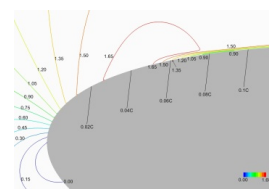
NACA0015翼まわりのキャビテーション解析
