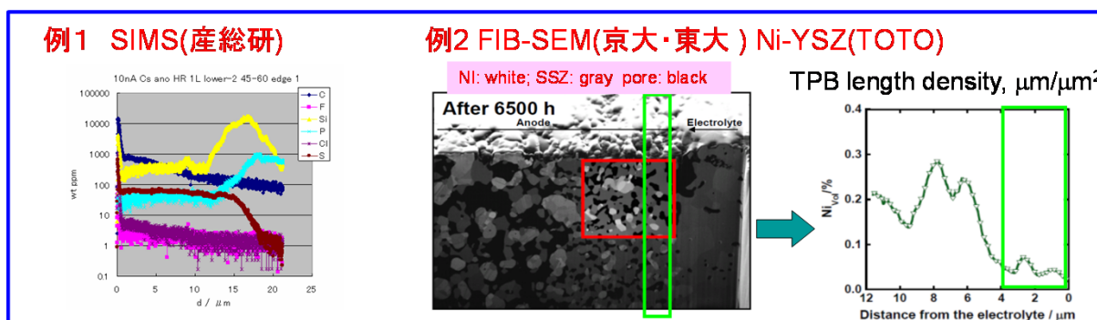
図1. TOTO製円筒縦縞形セルの劣化例(産総研のSIMS観測によって、P, Siが電気化学的活性点濃臭していること、京大・東大のFIB・SEM分析によって、活性点からNiが後退していることが明らかになった)
