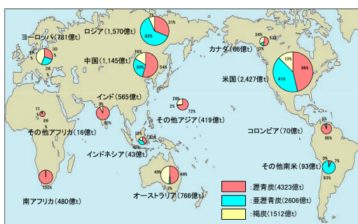
世界の石炭資源
