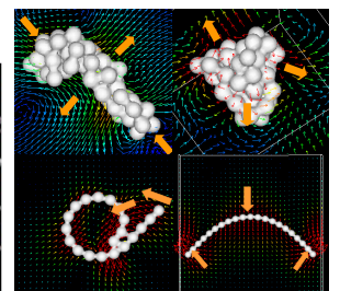
高分子鎖の凝縮転移時の流れ場の様子
