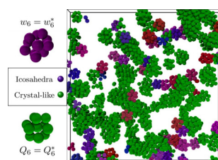
ガラス転移点近傍のコロイド過冷却液体における局所的な秩序化(実験)
