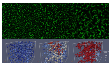
コロイド分散系におけるゲル化のメカニズム
