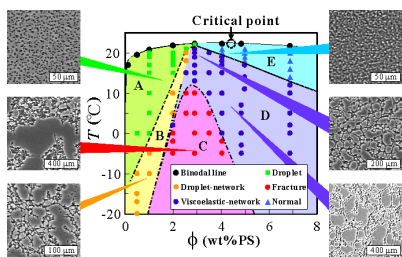
ポリスチレン-ジェテルマロナイト混合系で見られる様々な相分離パターンと相図
