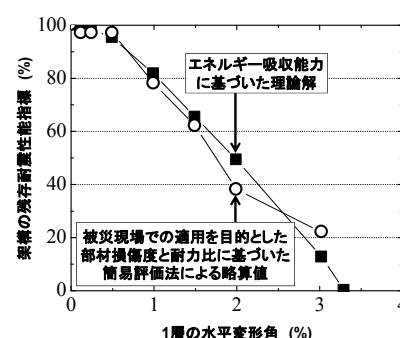
残存耐震性能評価(理論解 vs. 簡易評価法)
