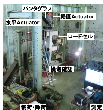
載荷実験の様子
