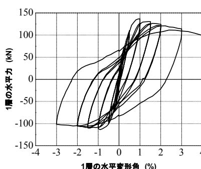
水平力と水平変形との関係
