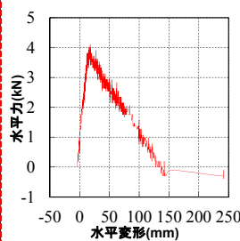
水平力と水平変形との関係
