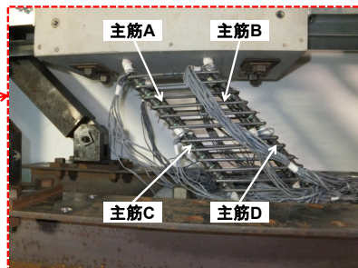
軸崩壊後の試験体の様子
