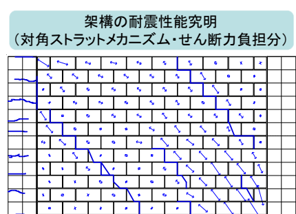
ブロック造壁の圧縮主歪度分布
