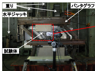
加力装置(正面図)
