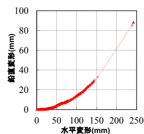
鉛直変形と水平変形との関係
