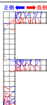
架構の損傷状態
