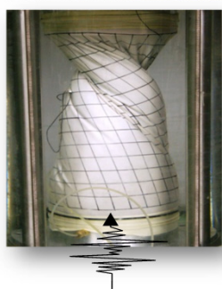
液状化発生前後の地盤強度の変化と中空供試体による液状化実験
