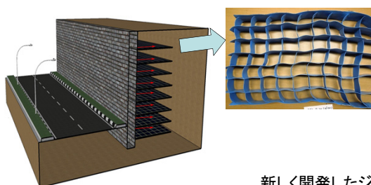
新しく開発したジオセルを用いた補強土擁壁の耐震性に関する研究 補強効果を引抜き試験と振動台模型実験で検討
